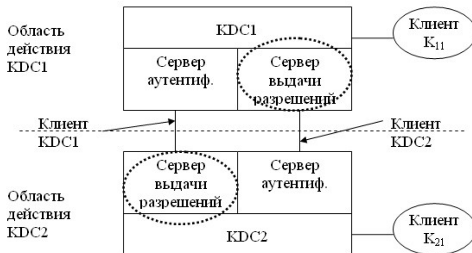
Рис. 2- Взаимодействие между Kerberos-областями
