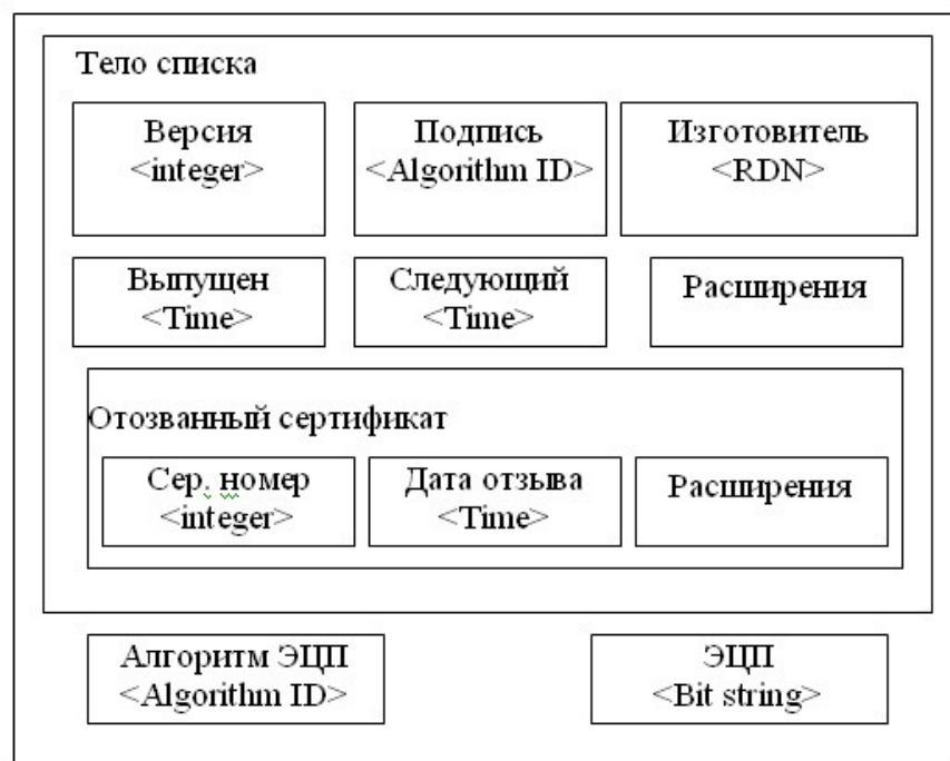
Рис. 5. Структура списка отозванных сертификатов
