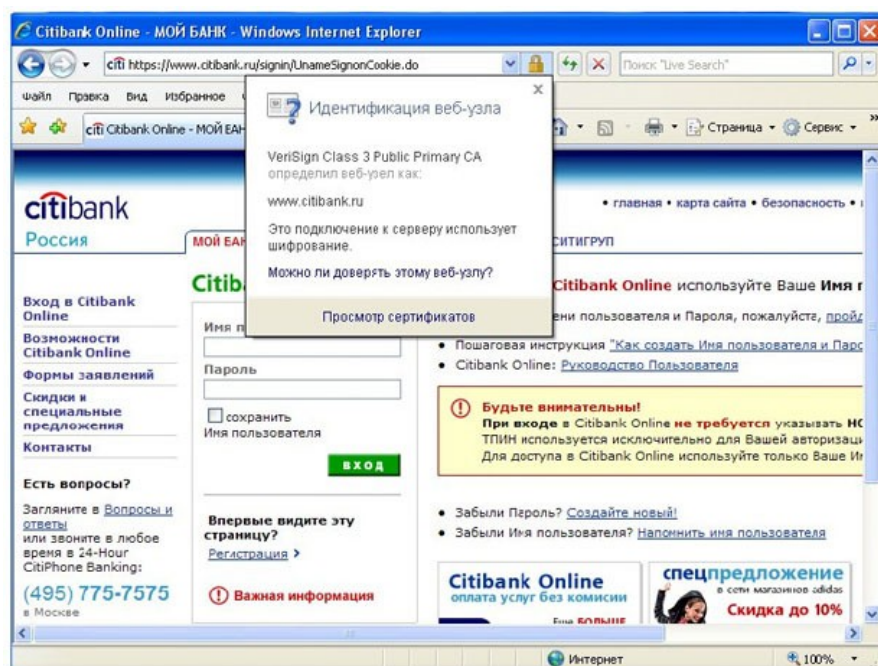
Рис. 1- Защищенное соединение
