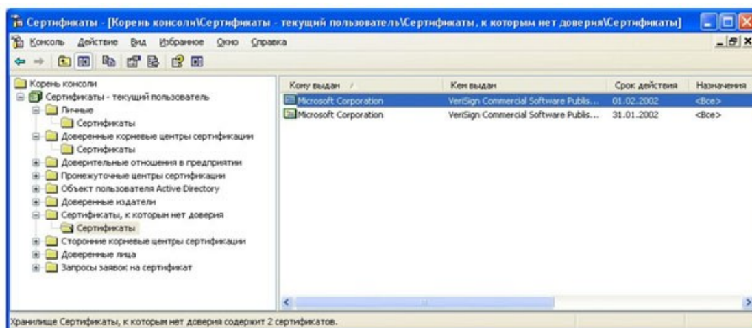
Рис. 4- Отозванные сертификаты
