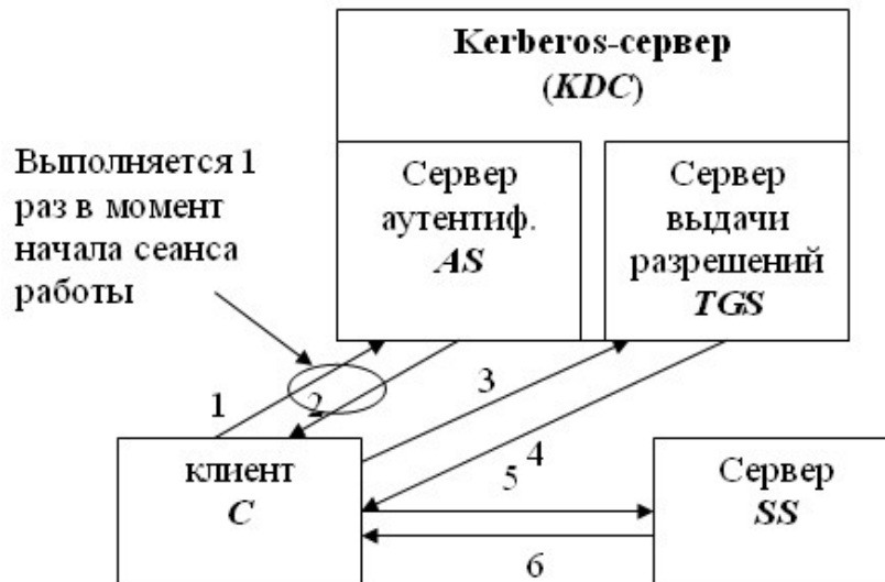
Рис. 1- Протокол Kerberos
