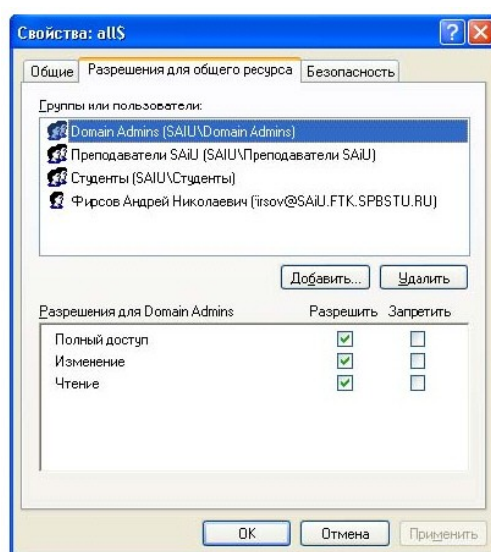
Рис. 6- Разрешения
