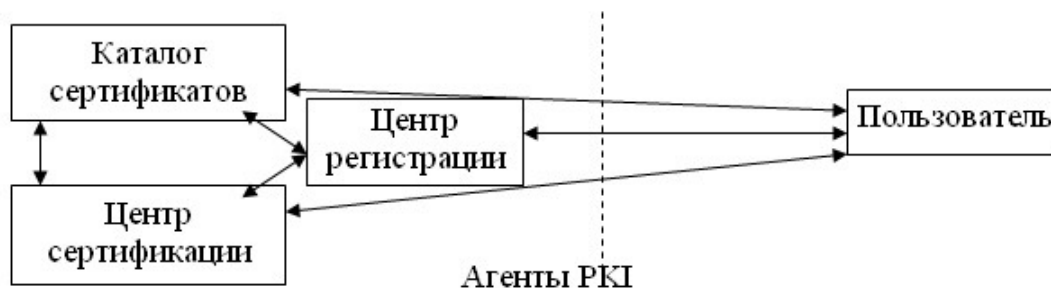
Рис. 2. Структура PKI
