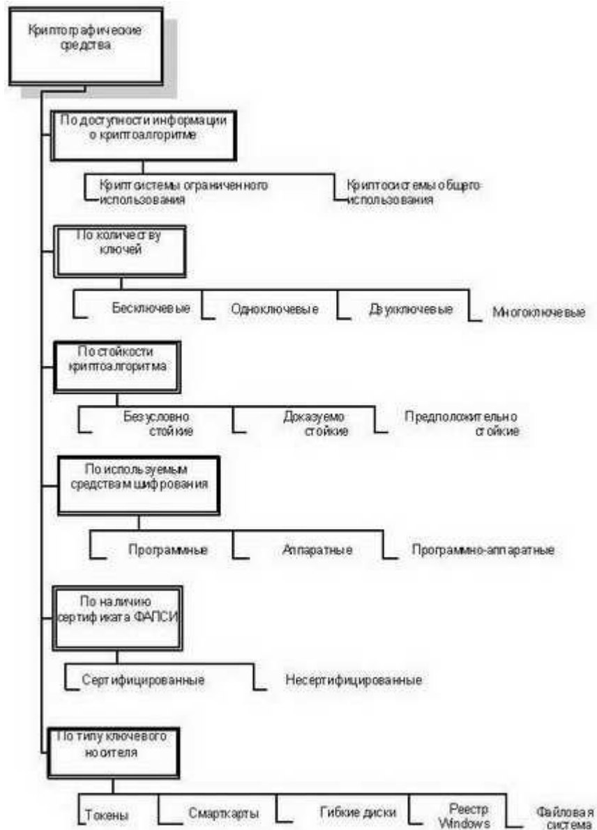
Рис. 7.3. Классификация криптосистем
