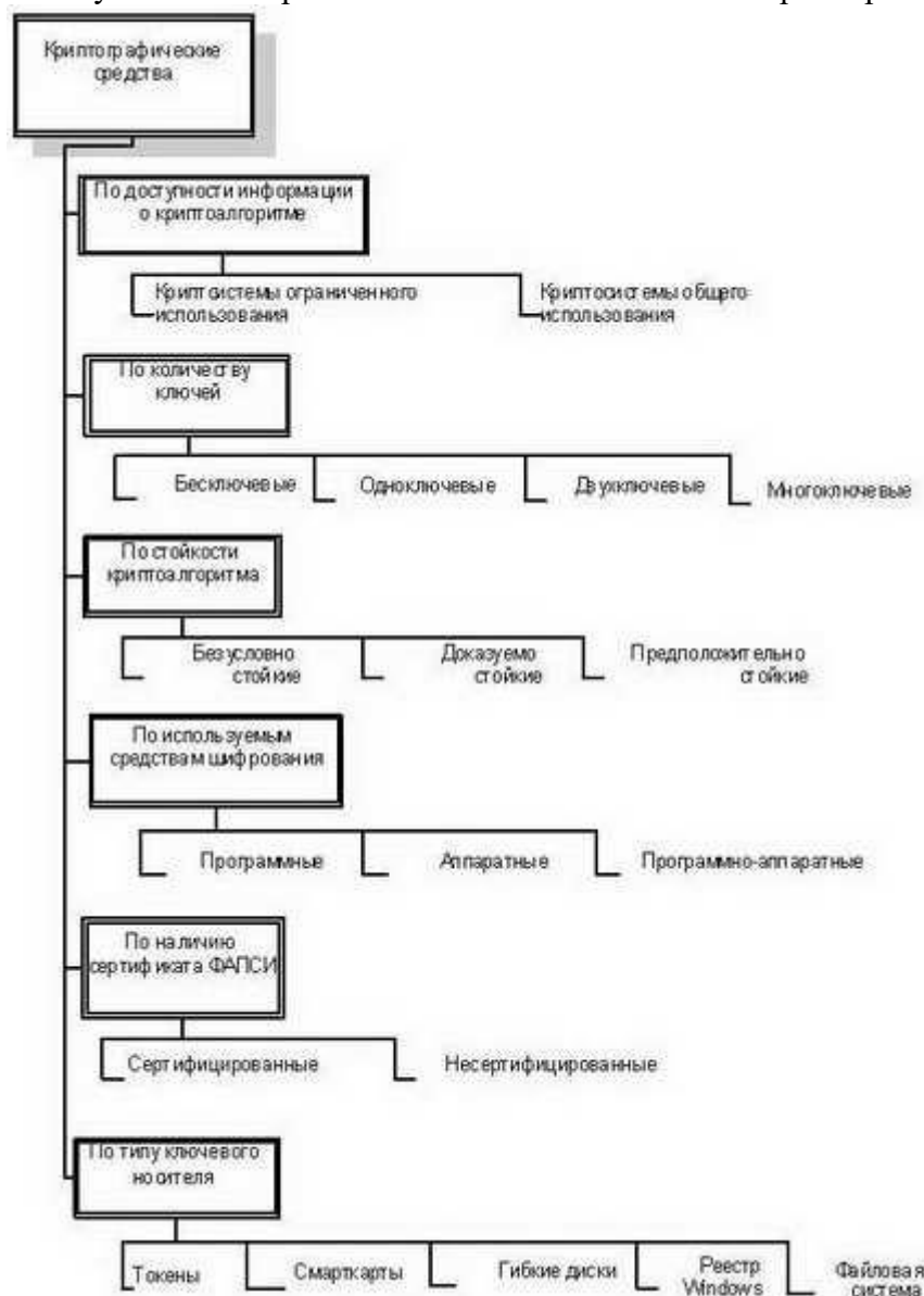
Рис. 7.3. Классификация криптосистем
