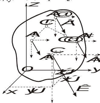
Рис. 1.37 Определение положения центра параллельных сил
