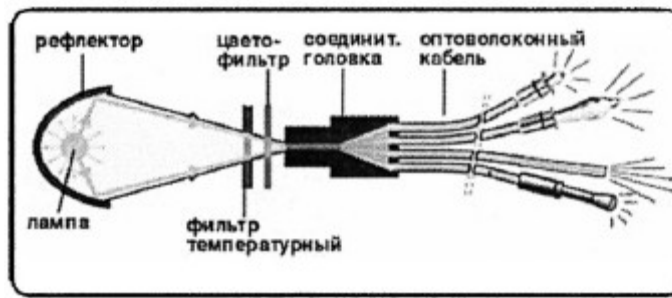
а) схема светильника
