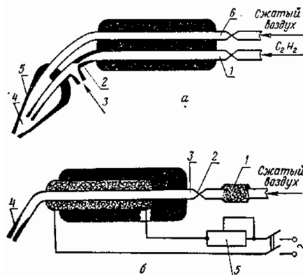
Рис. 2. Схема горелок для сварки термопластов горячими газами: а – газовая горелка ГП-1-56; б – газозлектрическая горелка
