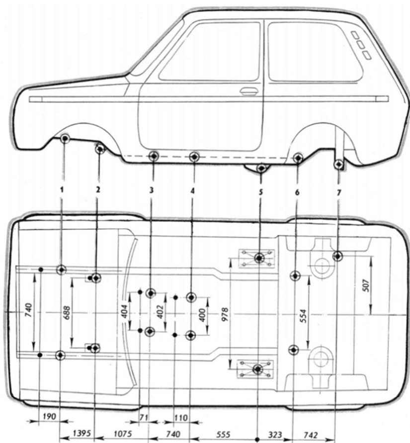
Рис. 11. Точки крепления двигателя и подвесок на кузове автомобиля модели ВА3-2121
