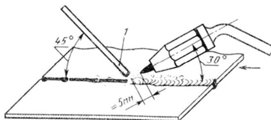
Рис. 5. Расположение горелки и припоя при пайке латунным припоем: I – порошковый флюс, нанесенный на конец припоя или прутка, покрытый флюсом
