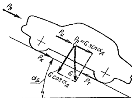
Рис 2.1 Силы, действующие на автомобиль при движении на подъем Сила тяги P_T представляет собой отношение момента M_T на полуосях к радиусу r ведущих колес при равномерном движении автомобиля:
