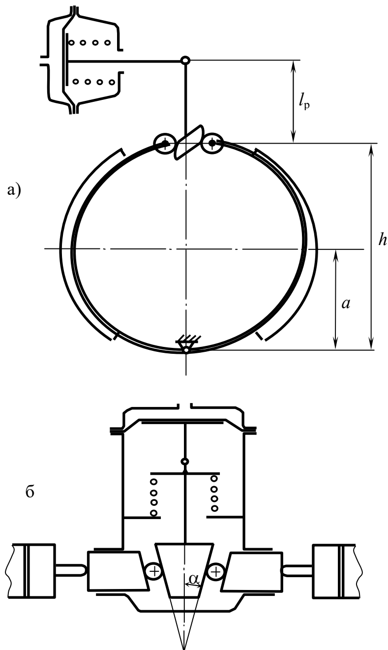
Рисунок 2.1 - Схемы тормозных механизмов: а – кулачковый; б - клиновйй.
