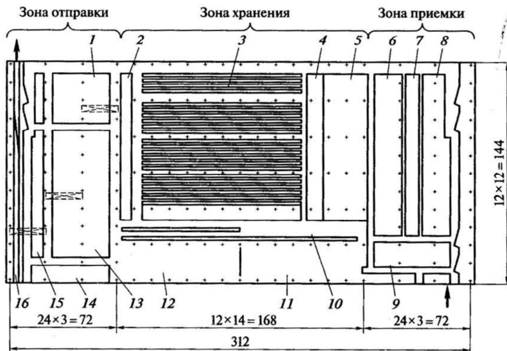
Рис. 9.7. Схема центрального склада запасных частей Волжского автозавода:
