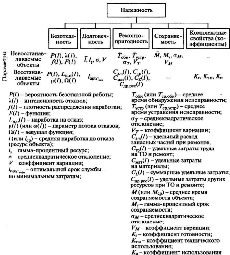
Рис. 3.9. Структура надежности
