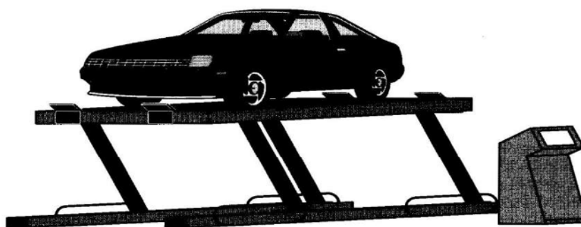
Рис. 5.12. Параллелограммный подъемник для легковых автомобилей
