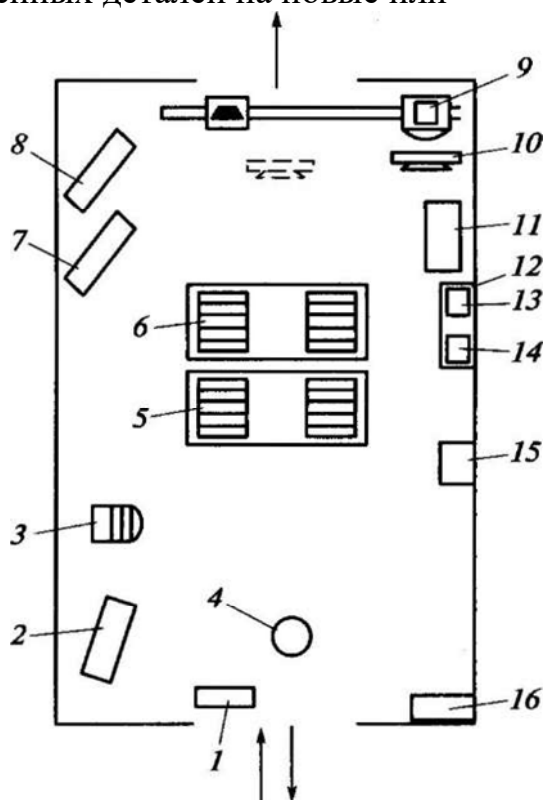
Рис. 7.6. Планировка поста диагностирования при ограниченных производственных площадях:
