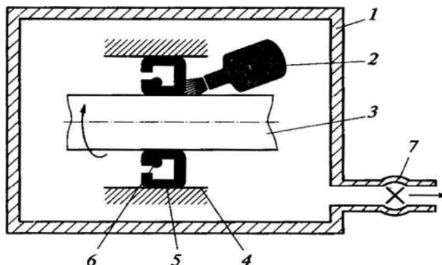
Рис. 3.5. Схема установки по изменению свойств резины:
