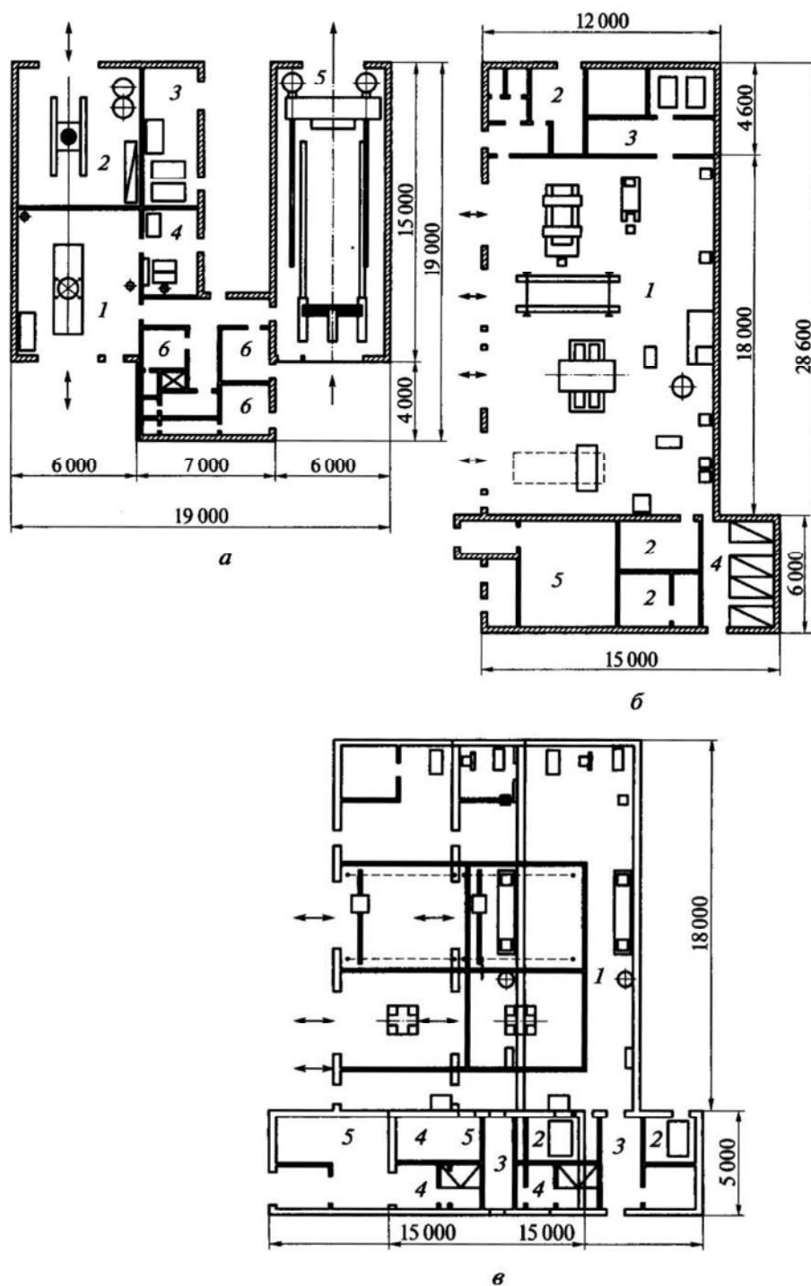
Рис. 4.5. Примеры планировок специализированных ремонтно-обслуживающих предприятий автосервиса:
