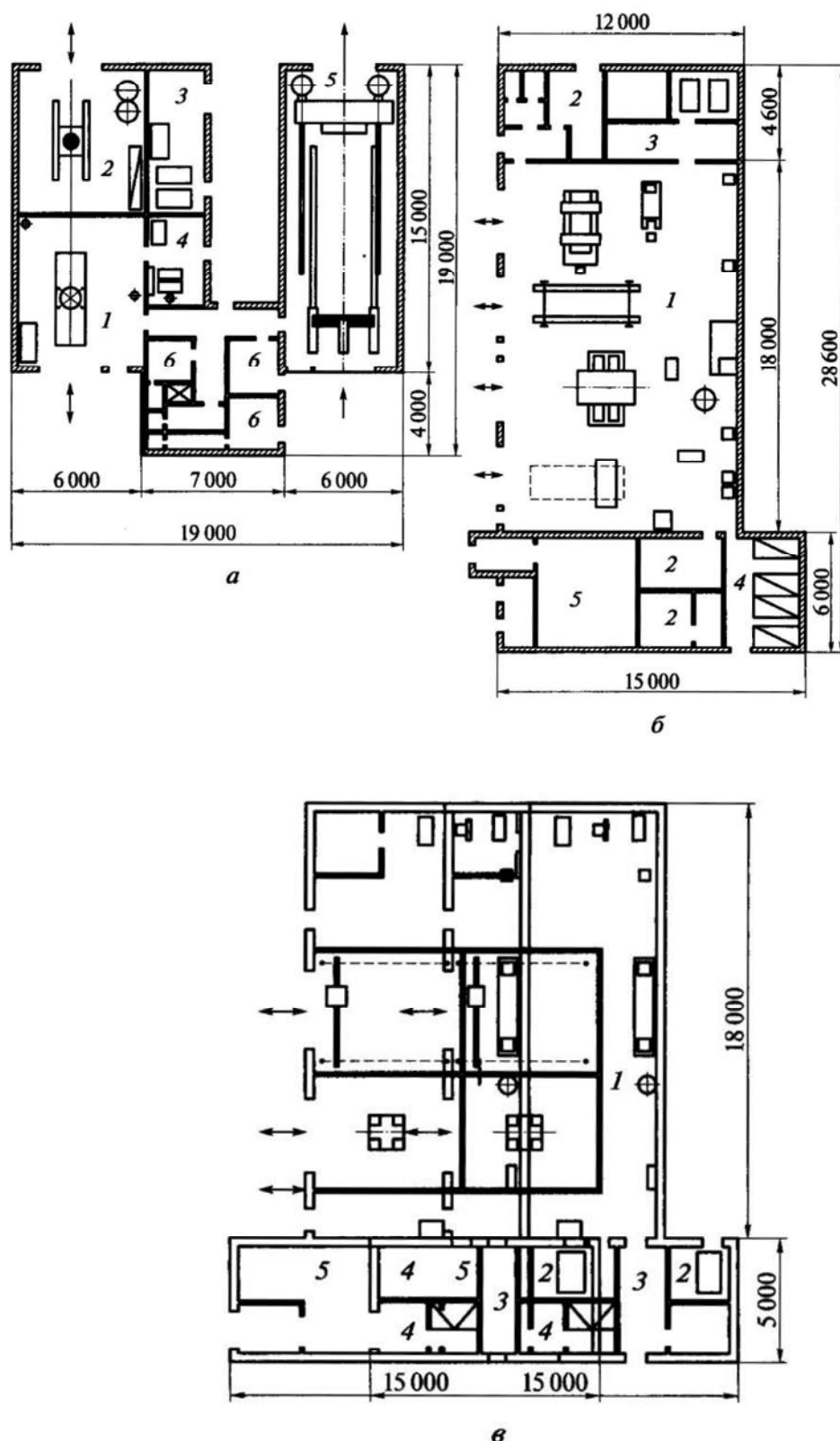
Рис. 4.5. Примеры планировок специализированных ремонтно-обслуживающих предприятий автосервиса:
