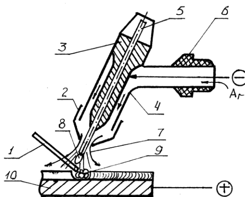
Рис.6. Схема электродержателя для аргонно-дуговой сварки: 1 - присадочный пруток; 2 - сопло; 3 - токоведущий мундштук; 4 - корпус; 5 - электрод; 6 - рукоятка; 7 - атмосфера защитного газа; 8 - сварочная дуга; 9 - ванна расплавленного металла; 10 - деталь
