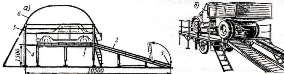
Рис. 5.4. Передвижные сборные эстакады: а - для легковых автомобилей; б - для грузовых автомобилей
