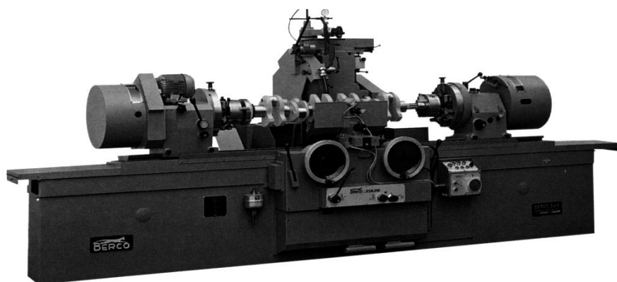
Рис. 3. Круглошлифовальный станок.
