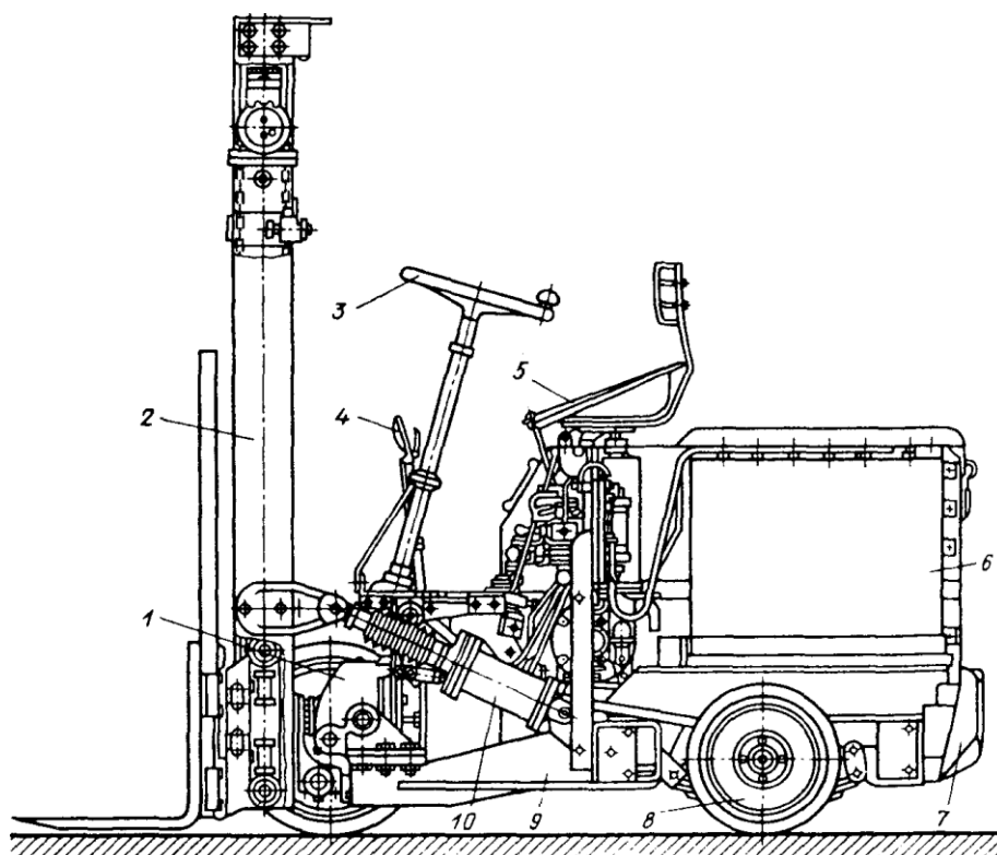
Рисунок 12. Устройство четырехколесного погрузчика:
