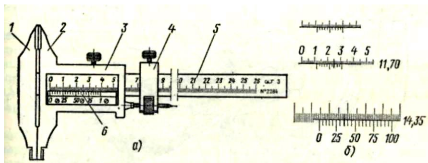
Рисунок 4. Штангенциркуль:
