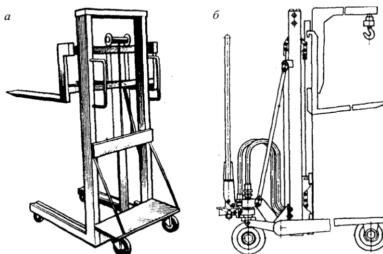
Рисунок 8. Ручная тележка-штабелер (а) и тележка-штабелер с безблочной консольной стрелой (б)
