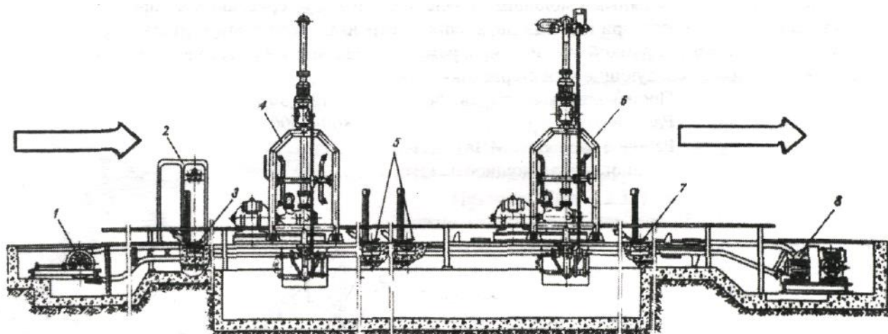
Рис. 15. Моечная установка мод. 1114с конвейером (вид сбоку): 1 - натяжная станция конвейера; 2 — аппаратный шкаф; 3, 5 и 7 - педали управления установкой и конвейером; 4 - секция предварительного обмыва; 6 - секция окончательного обмыва; 8 - приводная станция конвейера
