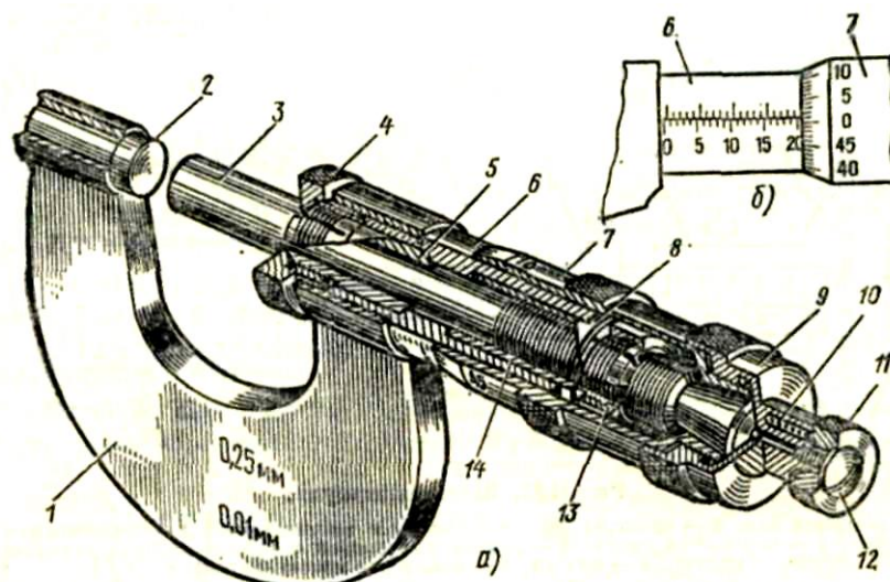
Рисунок 5. Микрометр:
