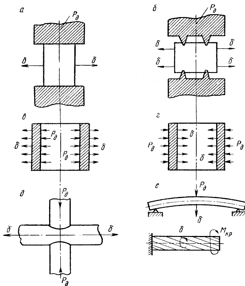
Рис. 5. Схемы восстановления деталей пластическим деформированием
