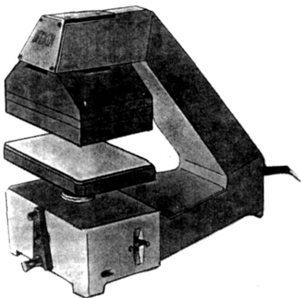
Рис. 13. Электровулканизатор для ремонта камер фирмы-экспортера «МОТОКОУ» (Прага, Чехия)
