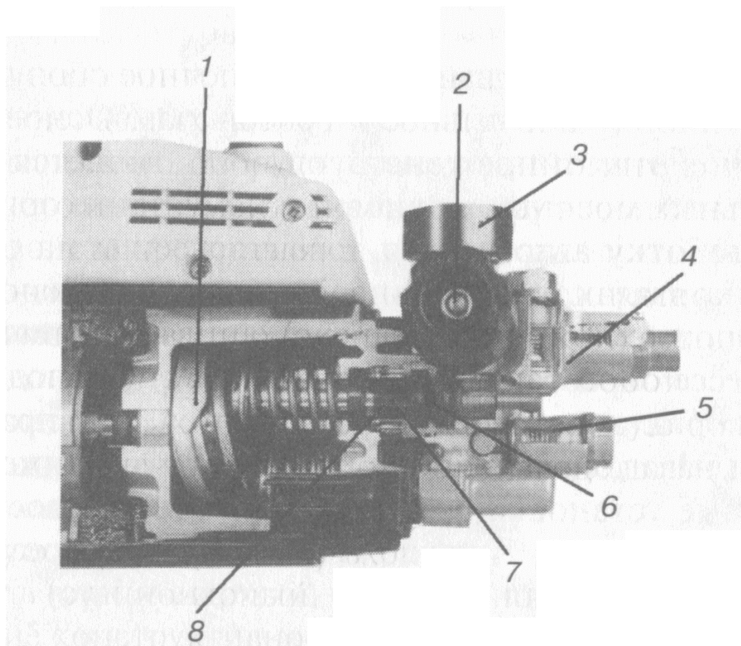
Рисунок 1.3 Насос высокого давления.
