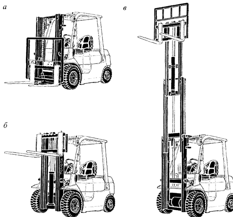
Рисунок 13. Электропогрузчики с различными типами мачт: а-VnSV;б-FV;в-FSV
