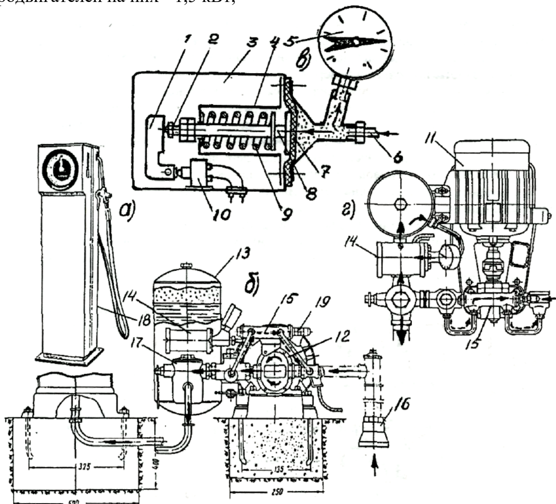
Рис. 3. Установка для раздачи масел для двигателей:
