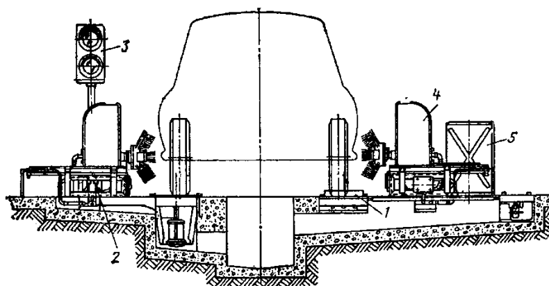
Рисунок 2.10 Установка для мойки колёс легковых автомобилей.
