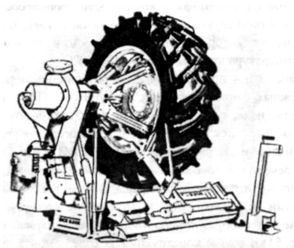
Рис. 11. Стенд для монтажа-демонтажа шин грузовых автомобилей с горизонтальным расположением силового цилиндра мод. S-208 фирмы «SICE» (Италия)
