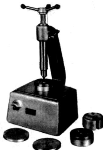
Рис.19. Аппарат электровулканизационный мод. 6134
