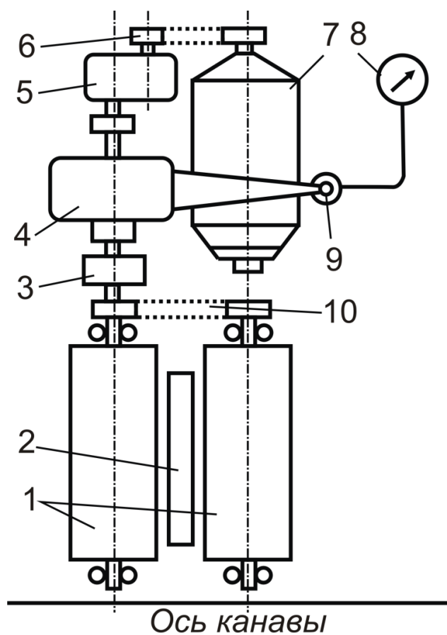
Рисунок 7.7. Схема роликового испытательного стенда RH-3000 (ПНР)
