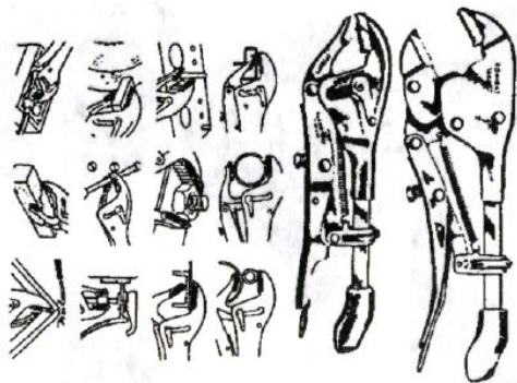
Рис. 5. Пассатижи с усилителем зажима деталей.
