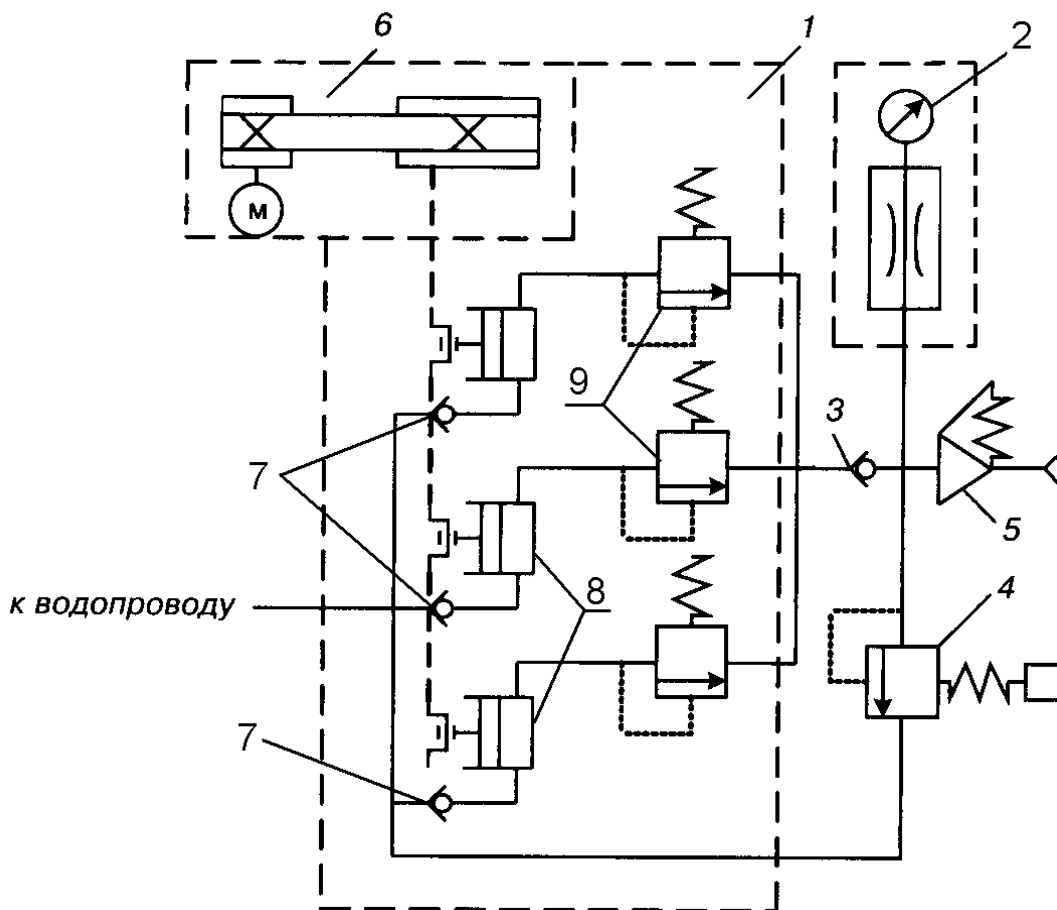
Рисунок 1.1 Типовая гидравлическая схема шланговой установки.
