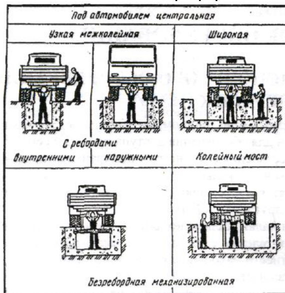
Рис. 2. Способы установки автомобилей на осмотровых канавах
