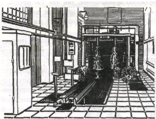
Рис. 6. Общий вид поточной линии мод. М-133
