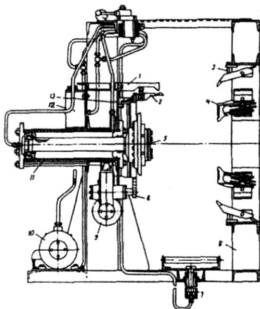
Рис. 5. Стенд для демонтажа и монтажа шин мод. Ш-509
