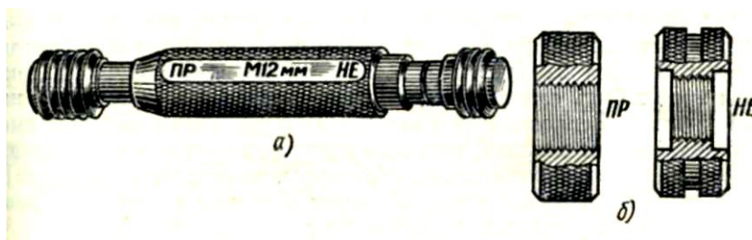
Рис. 12. Резьбовые калибры: а – предельная резьбовая пробка, б – нерегулируемые резьбовые кольца
