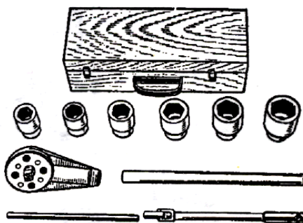
Рис. 3. Редуктор-усилитель крутящего момента с набором торцовых ключей
