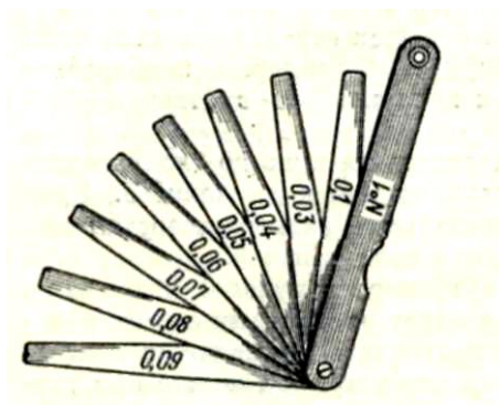
Рис. 9. Набор щупов
