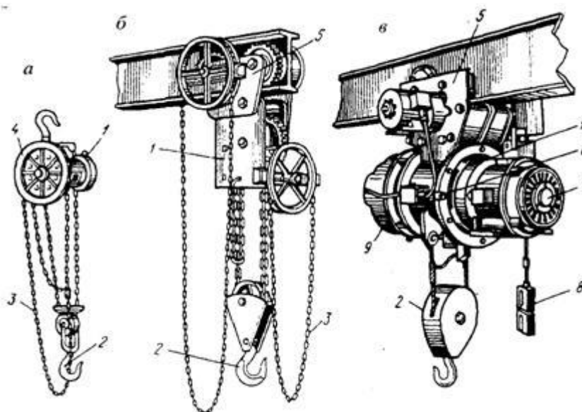
Рисунок 2 Тали ручные (а, б) и электрическая (в):
