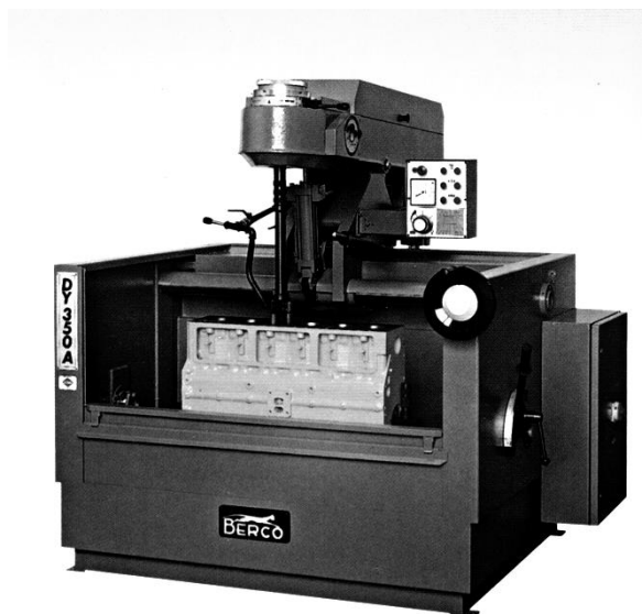
Рис. 2. Хонинговальный станок.
