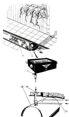
Рис. 3. Система комплексной заправки, смазки и слива отработанных масел
