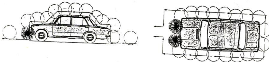
Рис. 14. Траектория движения щеток портальных установок
