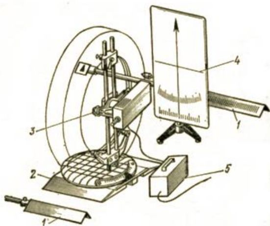
Рис. 7.6. Прибор «Оптиконт» для проверки углов установки управляемых колес легковых автомобилей мод. 2314 (ЧССР)
