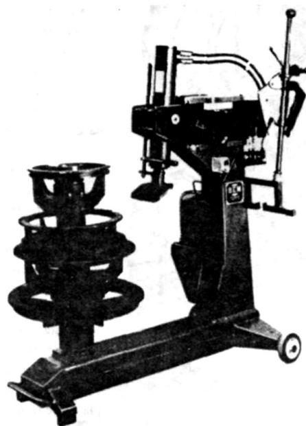
Рис. 12. Передвижной стенд для монтажа-демонтажа шин различного диаметра фирмы «BEM» (Франция)
