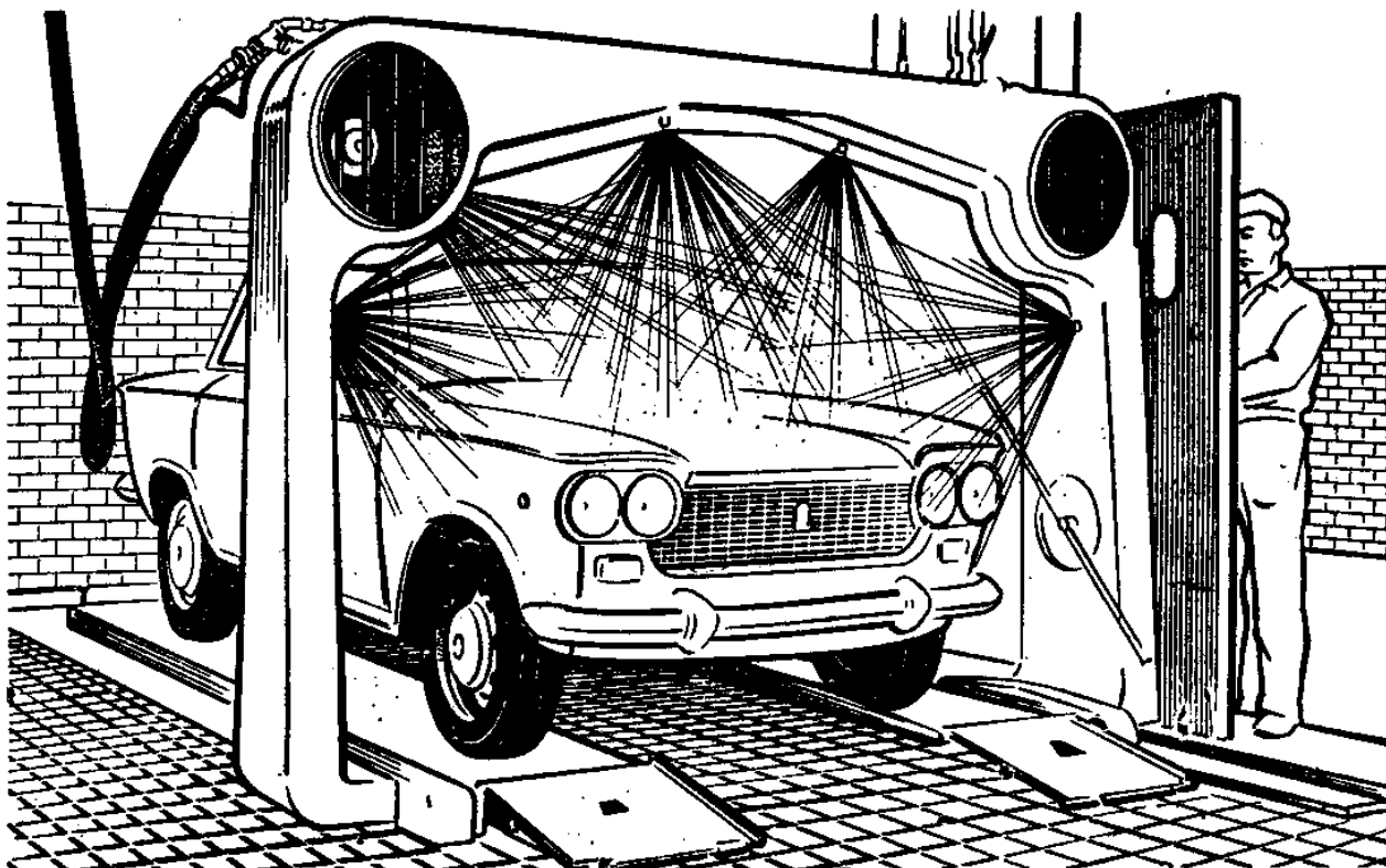
Рисунок 2.3 Портальная установка для струйной мойки наружных поверхностей кузова автомобилей
