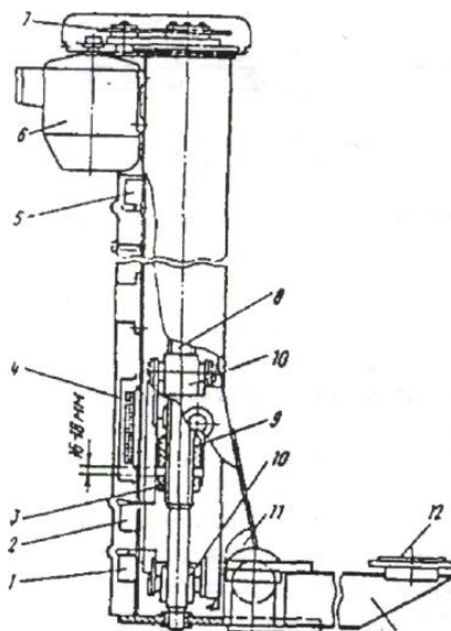
Рис. 7. Левая стойка двухстоечного подъемника с электро механическим приводом: 1 - аварийный выключатель; 2, 5 - концевые выключатели; 3 - страховая гайка; 4 - электроклемник; 6 - электродвигатель; 7 - цепная передача; 8 - рабочий винт; 9 - грузовая гайка; 10 - опора винта; 11 - каретка; 12-подхват; 13 - поворотная балка
