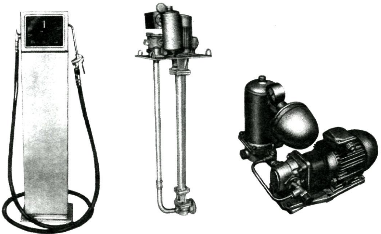
Рис. 6. Маслораздаточная колонка мод. 367М (а); погружная насосная установка мод. 3160 (б); стационарная насосная установка мод. 3106М (в)
