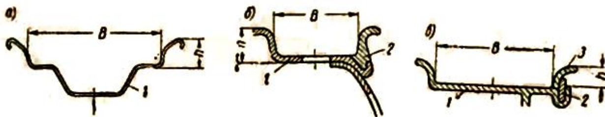
Рис. 1. Обода колес: B - ширина обода; h - высота закраины; 1 - обод; 2 - съемное разрезное бортовое кольцо, 3 - запорное бортовое кольцо
