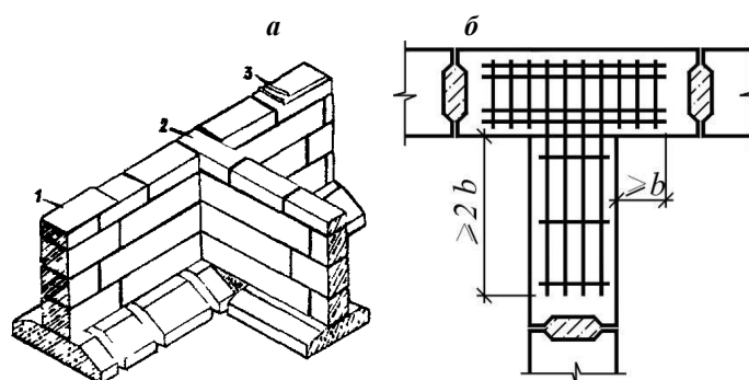
Рис. 2. Перевязка блоков продольных и поперечных стен подвала: а – перевязка блоков; б – усиление примыкания арматурными сетками; 1– выровненная поверхность стены подвала; 2 – перевязка блоков; 3 – гидроизоляция.
