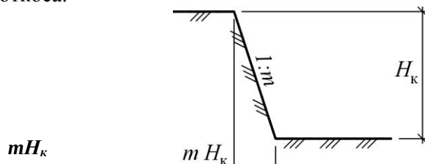
Рис. 3. Схема откоса
