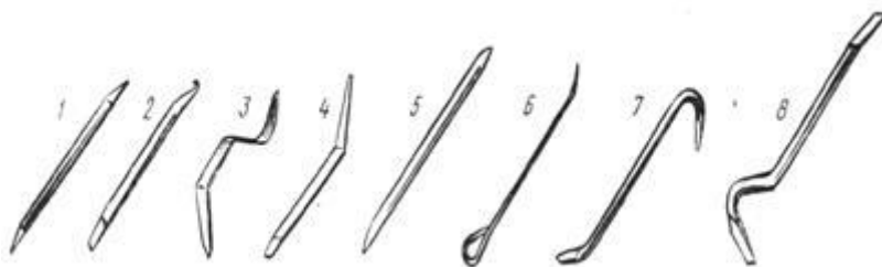
Рис.3. Рычаги и прижимы для исправления вмятин: 1-рычаг для исправления дефектов штамповки; 2-рычаг для рихтовки крыльев после окраски; 3-рычаг-прижим; 4-рычаг для исправления вмятин; 5-рычаг пластинчатый для исправления вмятин в труднодоступных местах; 6-рычаг для исправления разных дефектов; 7-рычаг для предварительной правки; 8-рычаг для устранения больших деформаций
