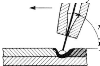
Рис. 11. Положение горелки при сварке в среде защитного газа
