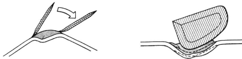
Рис. 2 - Нанесение шпатлевок на изогнутую поверхность
