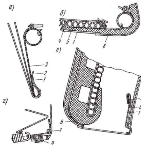
Рис. 3. Крепление обивки сидений: а - за зубцы металлических панелей остова сидения; б - к опорной сетке проволоочными скрепками; в - пружинной скрепкой к остоу спинки; г - шпагатом;
