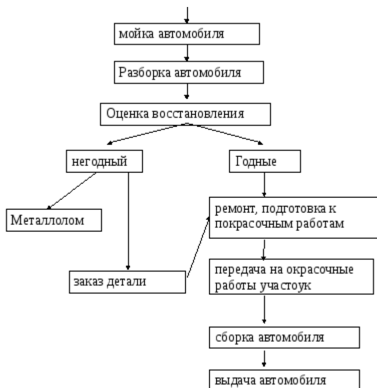
Рис. 1 - Общая схема производственного процесса на кузовном участке
