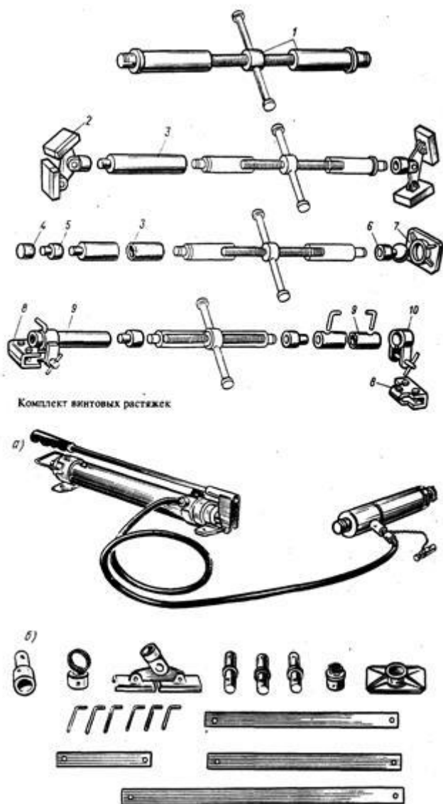
Рис.4. Оснастка для правки кузовов:
