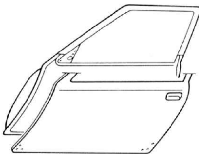
Рис. 20. Замена панели двери: зачистить следы точечной сварки фрезой, обрезать по линии разъема периферию панели двери, покрыть поверхность мастикой, закрепить новую панель, подогнать панель по месту и приварить точечной сваркой. Обеспечить герметичность внутренней полости
