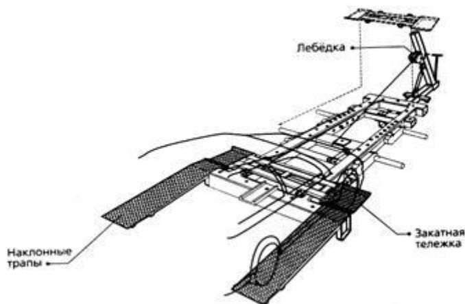
Рис 6. Установка автомобиля на стенд
