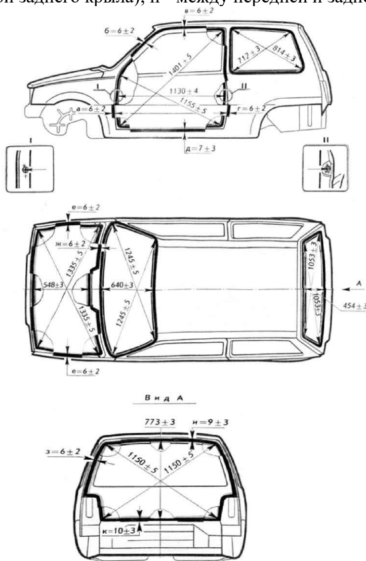
Рис. 9. Размеры проемов и зазоры спрягаемых деталей кузова автомобиля модели ВАЗ-1111
