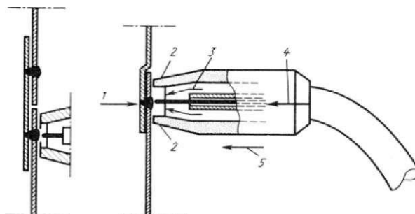
Рис. 12. Точечная сварка тонких листов, один из которых выполнен с накладной лентой, а другой с отбортовкой: 1 - сварная точка; 2 - мундштук; 3 - защитный газ; 4 - размотка с выдержкой времени; 5 - небольшое усилие сжатия
