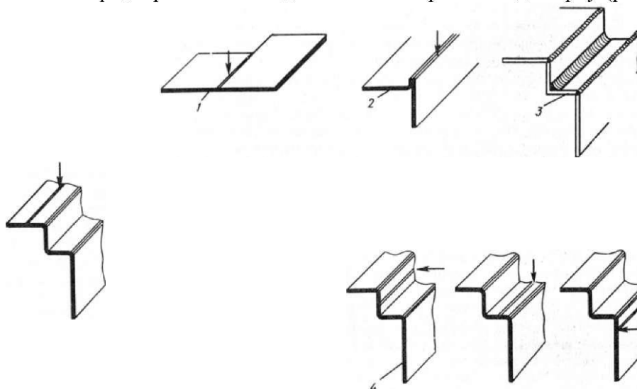
Рис. 6. Подготовка кромок тонких листов под сварку: 1 - сварка встык; 2 - сварка с отбортовкой кромки; 3 - сварка внутренних или наружных углов не подвергается рихтовке; 4 - хорошее расположение сварочного шва, позволяющего производить рихтовку
