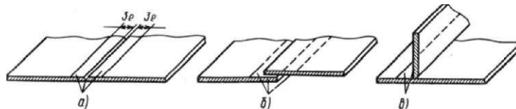
Рис. 4. Подготовка кромок к пайке латунным припоем: а - участки, зачищенные до металла; б и в - зачистка до чистого металла
