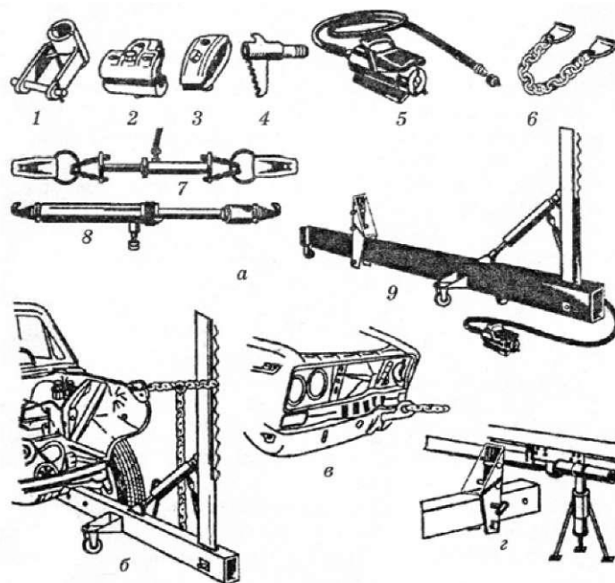
Рис. 17. Приспособления для выполнения правки деформированного участка кузова: а -комплект приспособления для устранения перекосов и перегибов; б, в и г - использование приспособлений при правке; 1 - оправка для вытягивания вогнутых деталей; 2 и 3 -самозакрепляющиеся гидравлические зажимы; 4 - оправка с зубцами для захвата выпрямляемой панели; 5 -насос; 6 -двойной захват; 7, 8 -натяжной цилиндр; 9 -фиксирующее устройство
