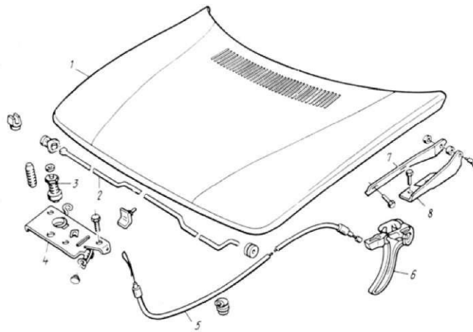
Рис. 19. Капот двигателя автомобиля с механизмом открывания: 1 -капот; 2 -тяги; 3 -отпирающий палец; 4 -замок; 5 -трос капота; 6 - рукоятка открывания капота; 7 и 8 -шарниры
