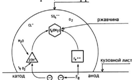
Рис. 1. Схематичное изображение процесса коррозии
