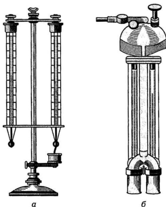
Рис. 3.1. Психрометры:
