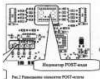
Рис.2 Размещение элементов POST-платы
