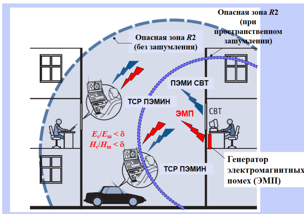
1. Для исключения перехвата побочных электромагнитных излучений по электромагнитному каналу используется пространственное зашумление , схема представлена на рисунке.
