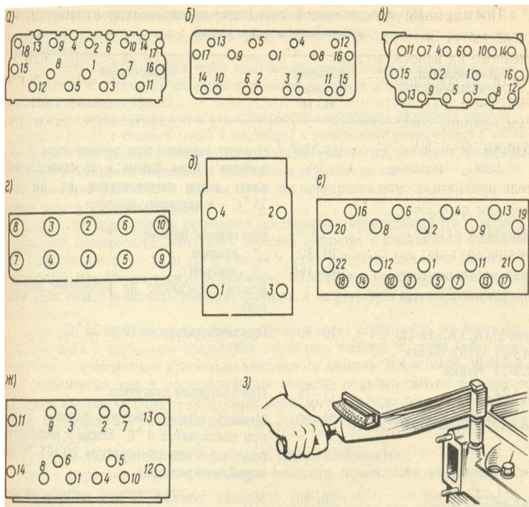
Последовательность затяжки гаек крепления головок цилиндров двигателей а – ГАЗ-53-12, -66-11,-14 «Чайка»; б - ЗИЛ-130, Урал-375Д, автобусы ЛиАЗ-677, ПАЗ-695Н, -699Р; в – МАЗ-5335; г – ГАЗ-24, -3102 «Волга»; д – КамАЗ -5320; е – ЗИЛ-4331; ж – Икарус-260; з – торцовый ключ с динамометрической рукояткой.
