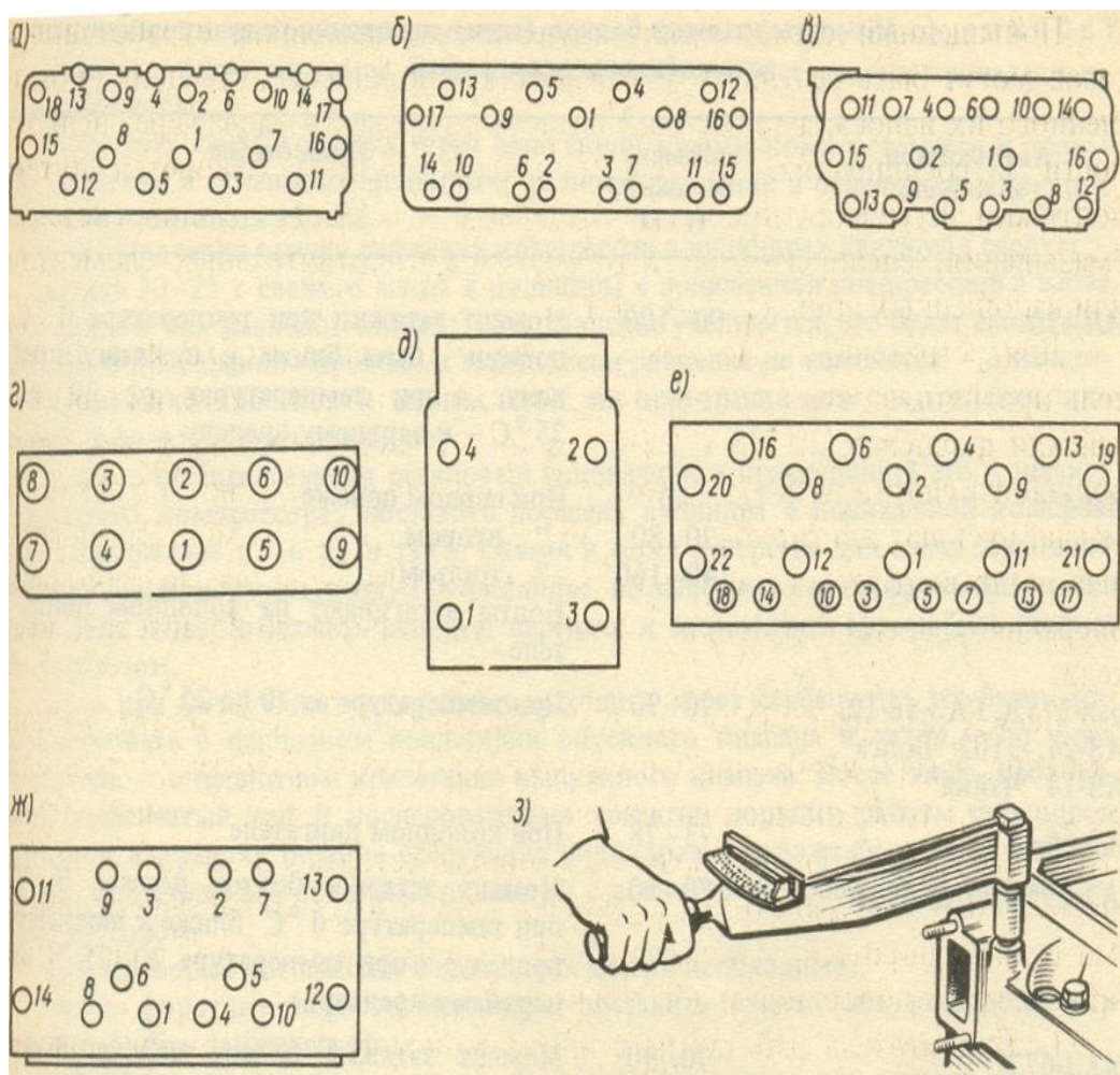
Последовательность затяжки гаек крепления головок цилиндров двигателей а – ГАЗ-53-12, -66-11, -14 «Чайка»; б - ЗИЛ-130, Урал-375Д, автобусы ЛиАЗ-677, ПАЗ-695Н, -699Р; в – МАЗ-5335; г – ГАЗ-24, -3102 «Волга»; д – КамАЗ -5320; е – ЗИЛ-4331; ж – Икарус-260; з – торцовый ключ с динамометрической рукояткой.
