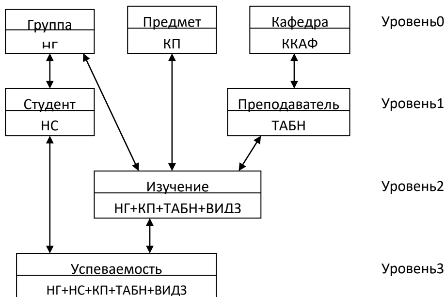
Рисунок 7.6 - Информационно-логическая модель предметной области "Учебный процесс"
