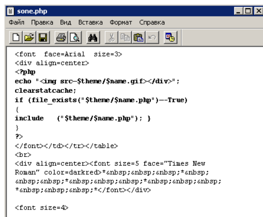
Рисунок 7.8 - Программа на PHP (выделена полужирным) в тексте web-страницы
