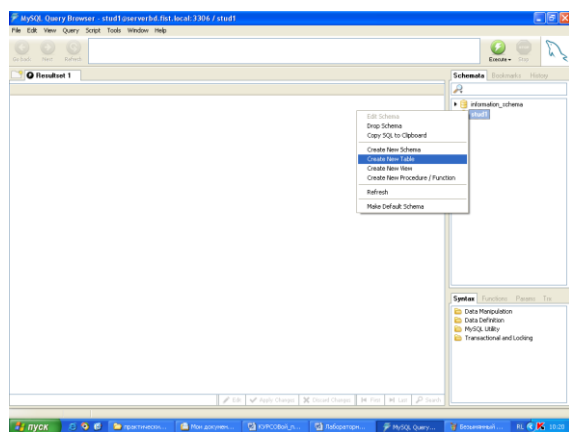
Рисунок 7.11 - Создание новой таблицы в MySQL
