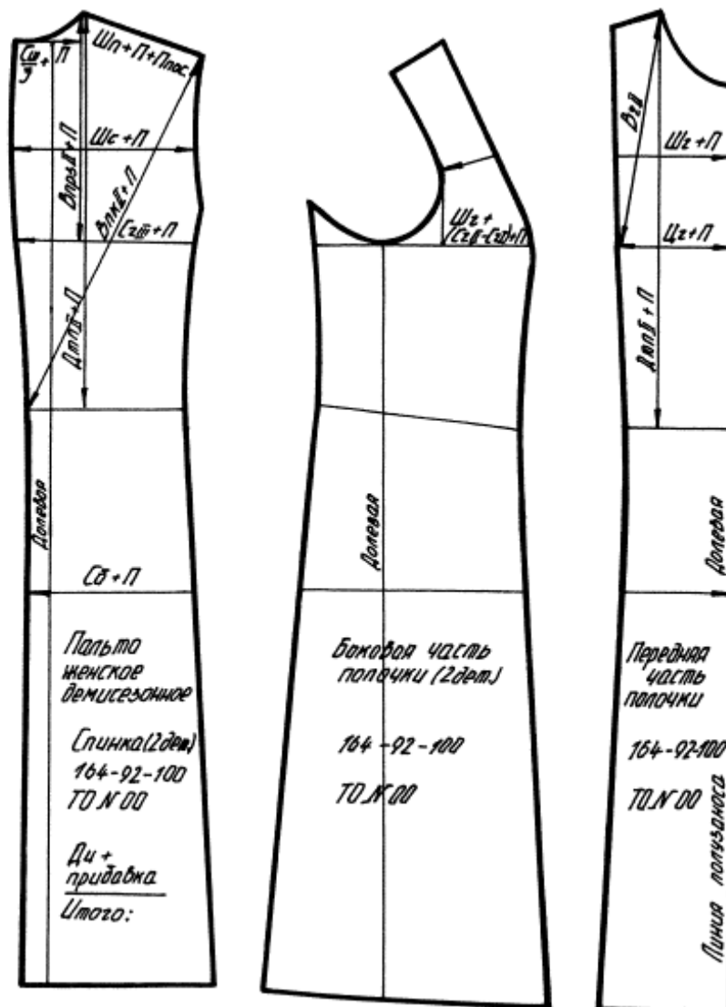
Рис. 17.5. Рабочие чертежи лекал базовых конструкций
