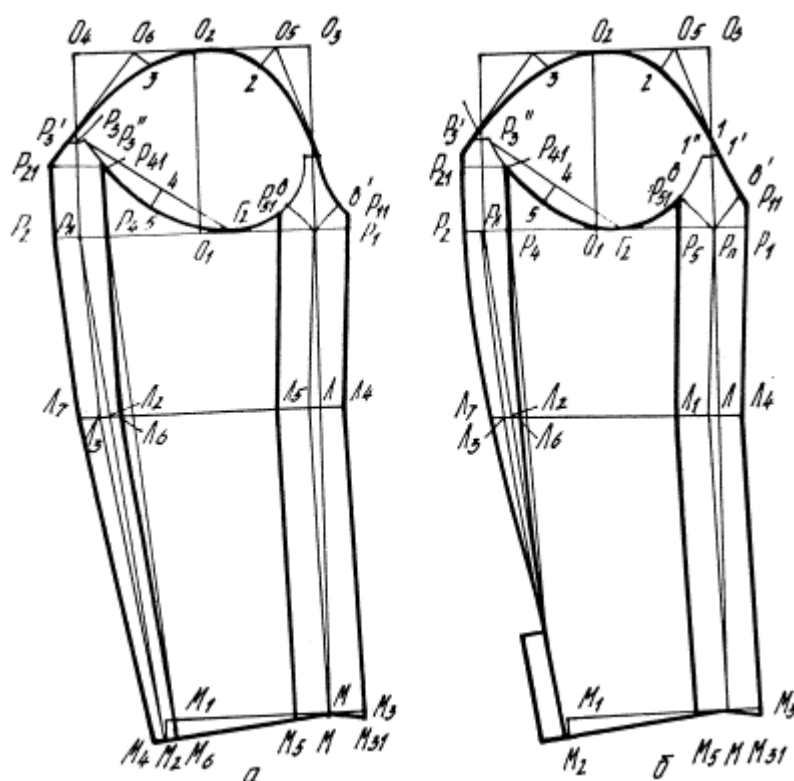
Рис. 5.3. Варианты конструкции двухшовного втачного рукава
