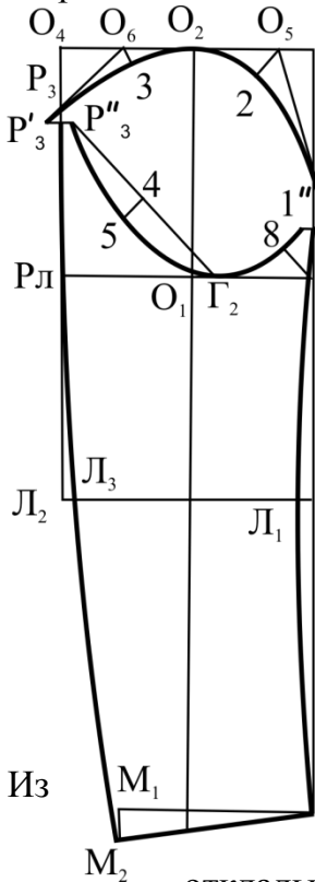
Рис. 12.2. Чертеж конструкции основы втачного рукава
