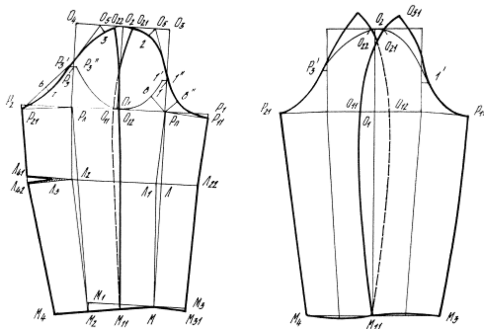
Рис. 5.6. Варианты конструкции рукавов с верхним срезом
