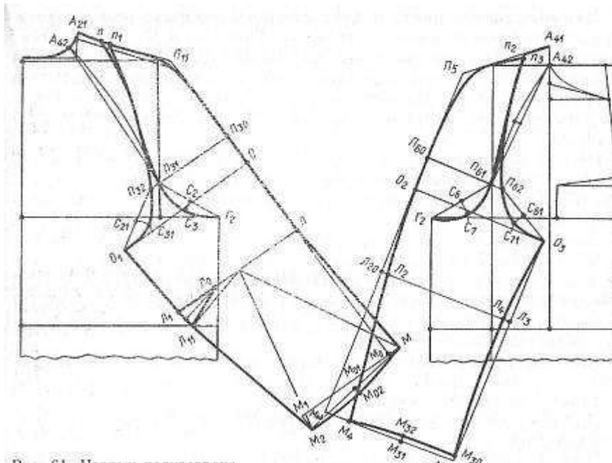
Рис. 8.4 Чертеж конструкции передней и задней части рукава покроя полуреглан
