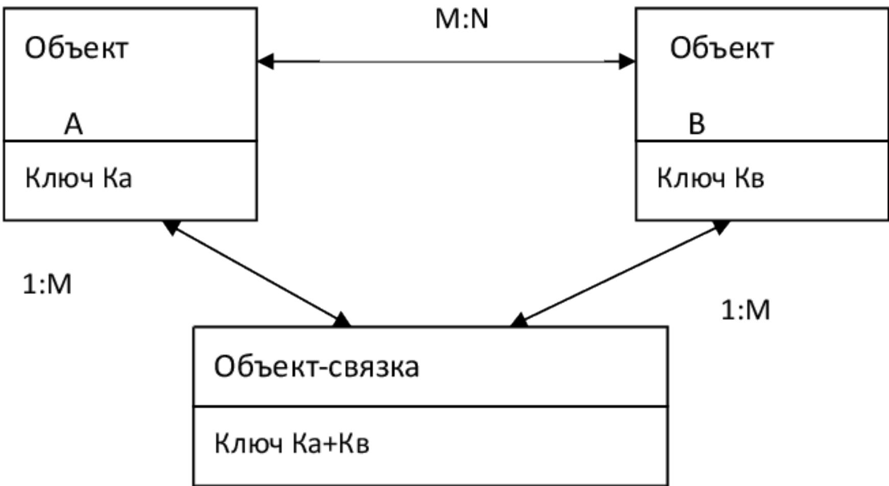
Рисунок 7.5 - Преобразование связи типа M:N через объект-связку.
