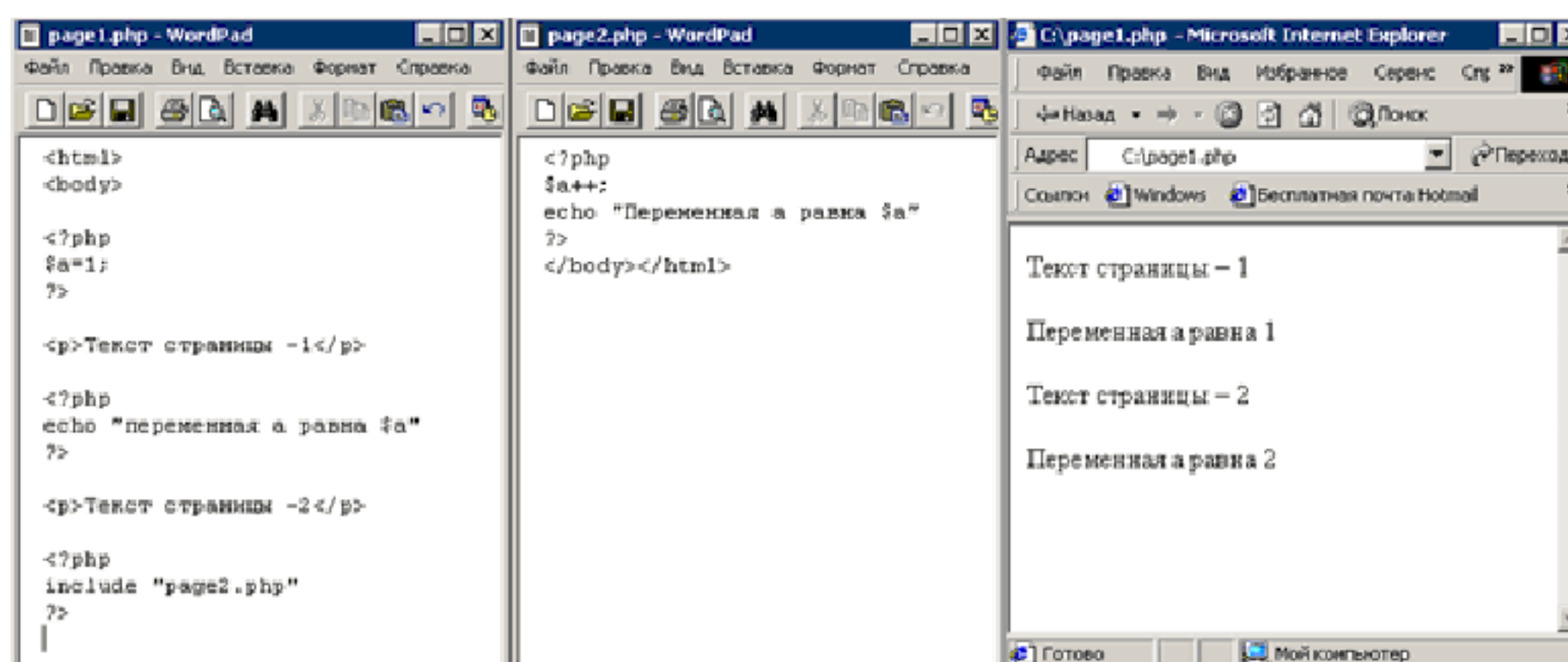
Рисунок 7.9. - Пример PHP-кода
