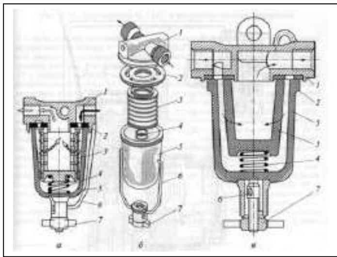
Рис. 7.3. Фильтры тонкой очистки топлива двигателей ЗМЗ-53 и ЗИЛ-130:
