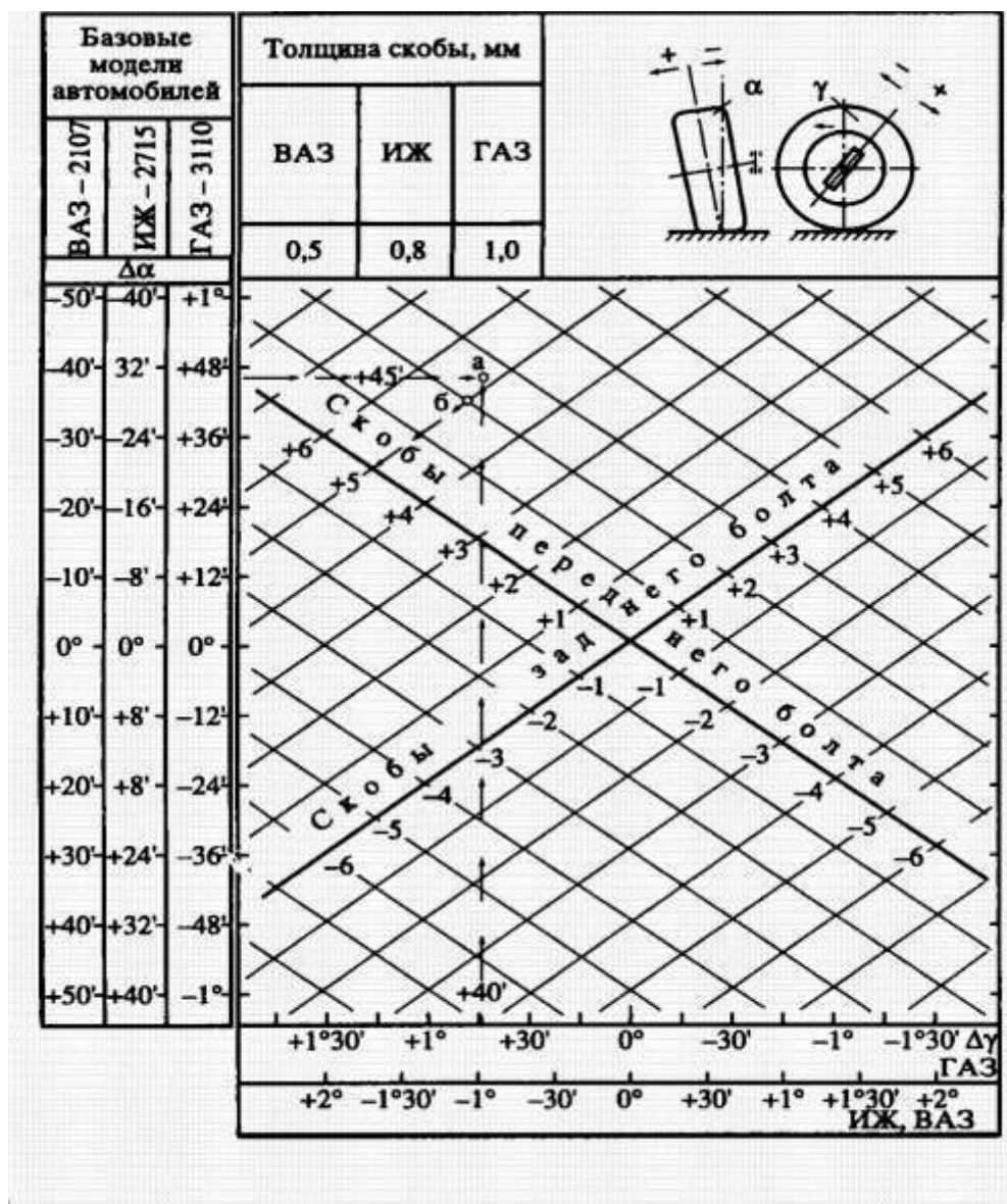
Рисунок 27 – Номограмма выбора технологических воздействий при совместной регулировке углов развала \alpha и продольного наклона оси поворотов \gamma
