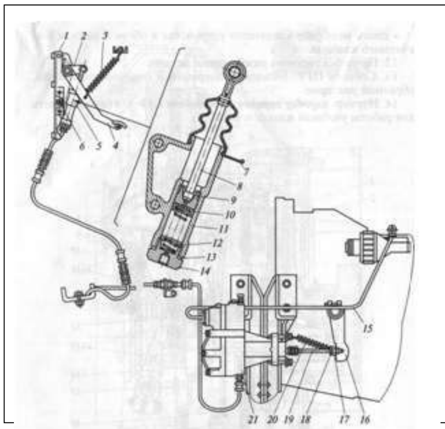
Рис. 4. Пневмогидравлический усилитель привода сцепления семейства КамАЗ:
