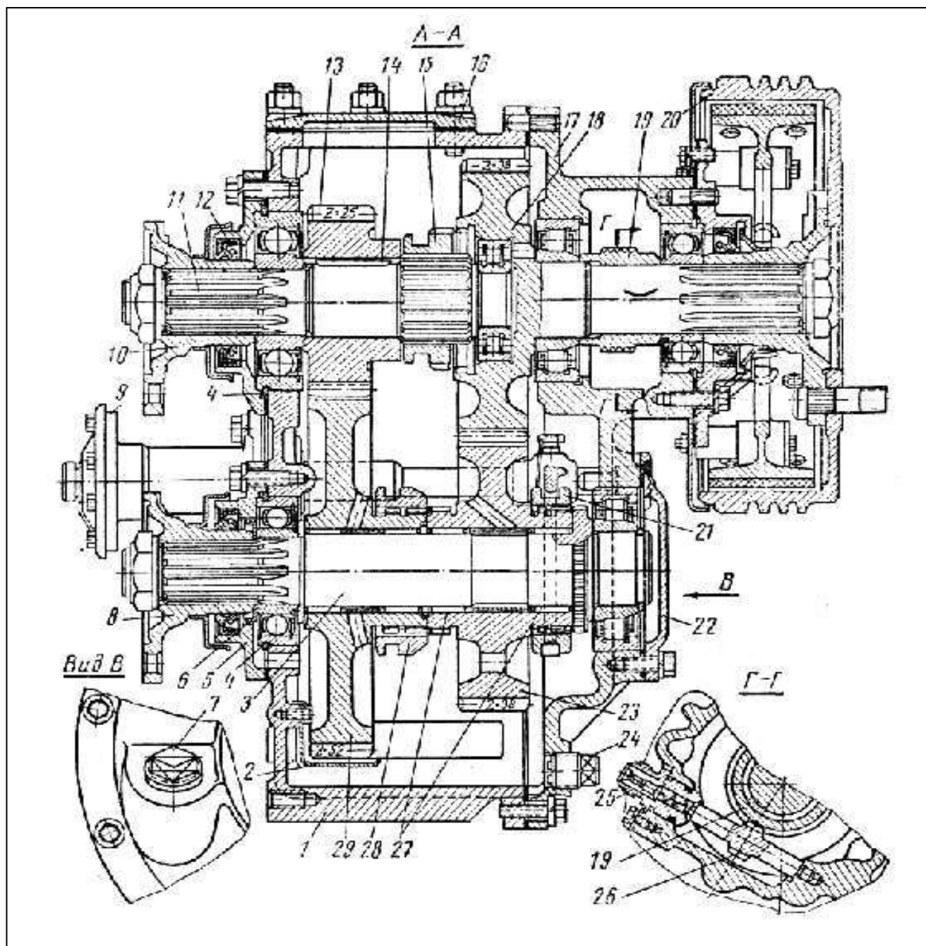
Рисунок 1 Устройство раздаточной коробки: 1 - картер раздаточной коробки; 2 - маслонаправляющий лоток; 3 - вал привода переднего моста; 4 - стопорное кольцо; 5 - крышка; 6 -маслоотгонная шайба; 7 - контрольно-заливная пробка; 8 - фланец привода переднего моста; 9 - пневматическая диафрагменная камера включения привода переднего моста; 10 - фланец первичного вала;
