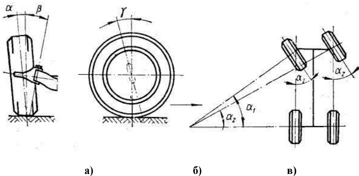
а) угол развала колеса и угол поперечного наклона шкворня; б) угол продольного наклона шкворня; в) углы поворота колес при повороте автомобиля
