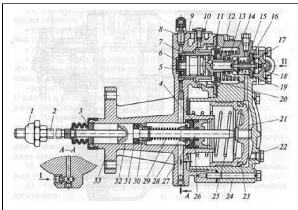
Рис. 5. Пневмогидравлический усилитель привода сцепления в автомобилях семейства КамАЗ:
