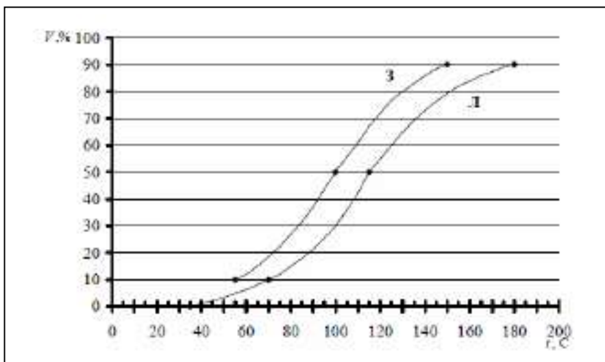
Рис. 4. Кривые испаряемости стандартных бензинов.
