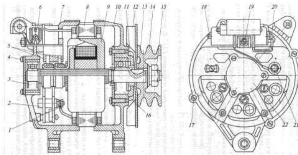
Рис. 12.2 Генераторная установка Г-237-В
