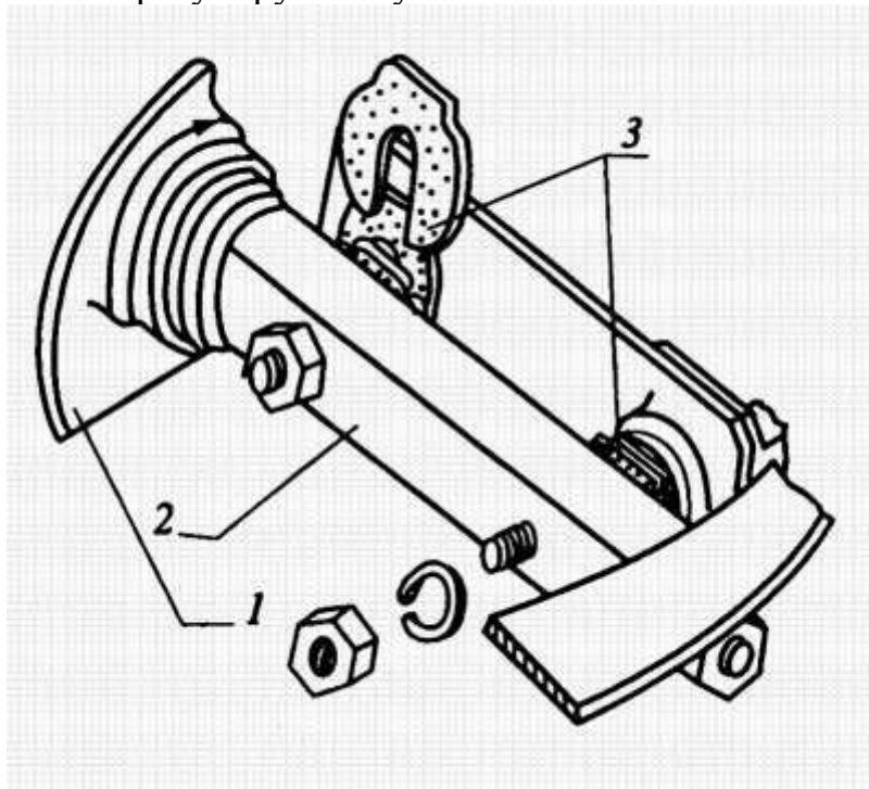
Рисунок 26 – Регулировка углов колес автомобиля с рычажной подвеской
