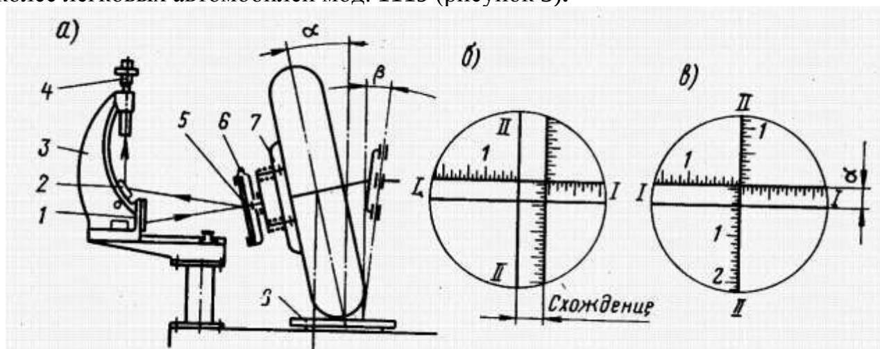
а) схема работы стенда; б, в – разметка линзы объектива
