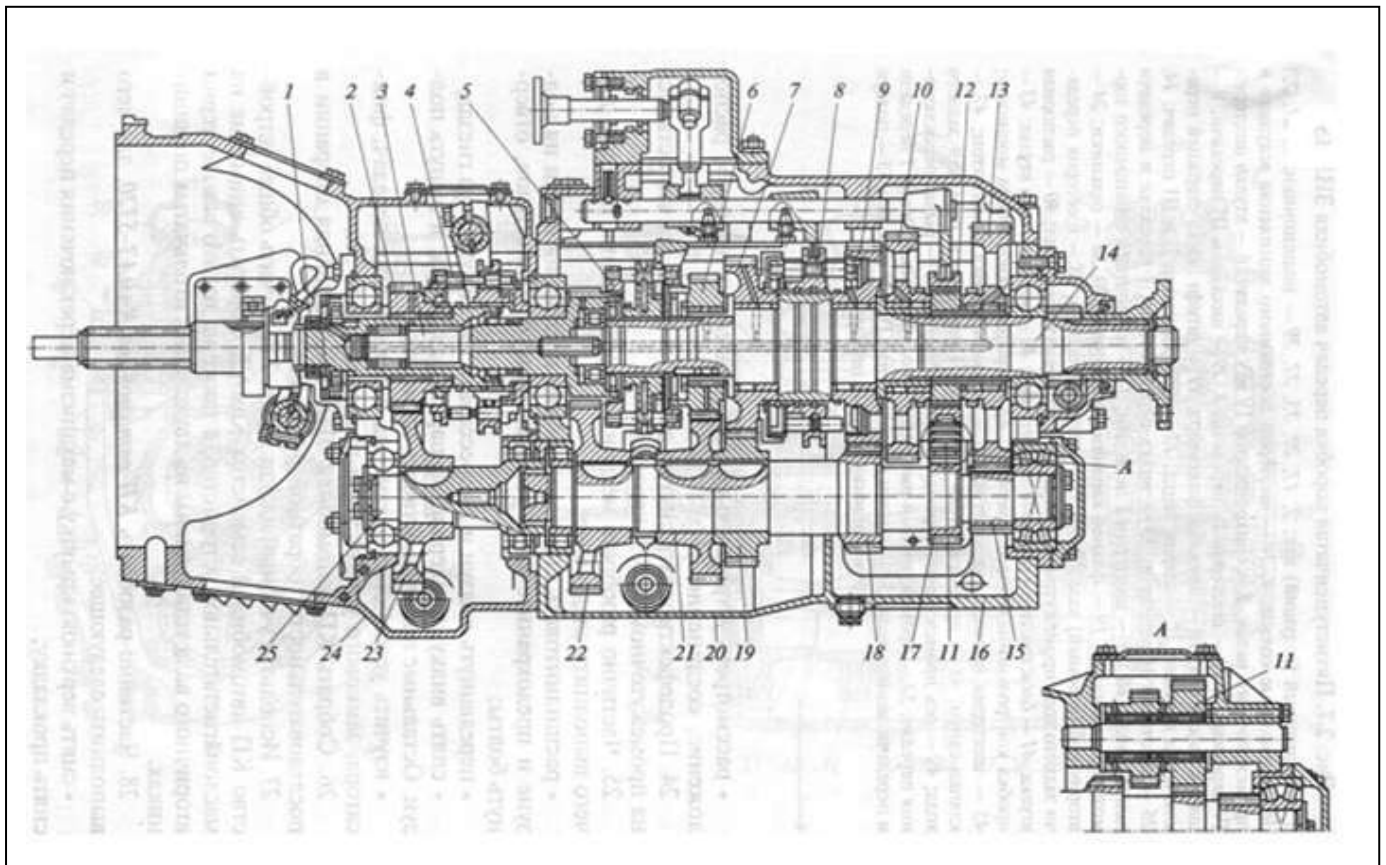
Рис. 3 Коробка передач автомобиля КамАЗ:
