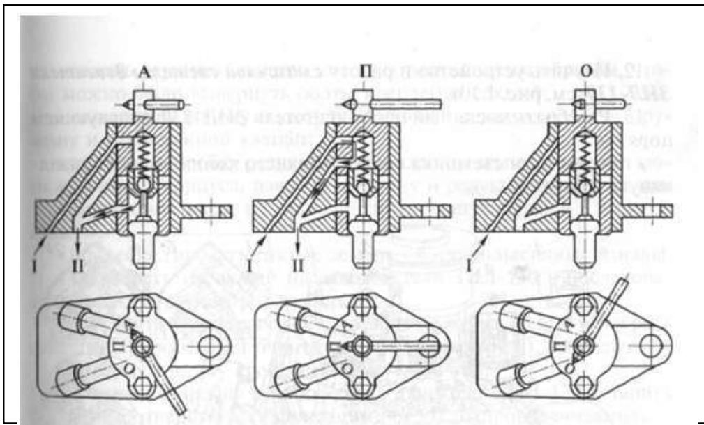
рис. 5.4. Положения (А, В, О) выключателя гидромукфы привода вентилятора: I – подача масла из смазочной системы двигателя; II – подача масла в гидромукфу.
