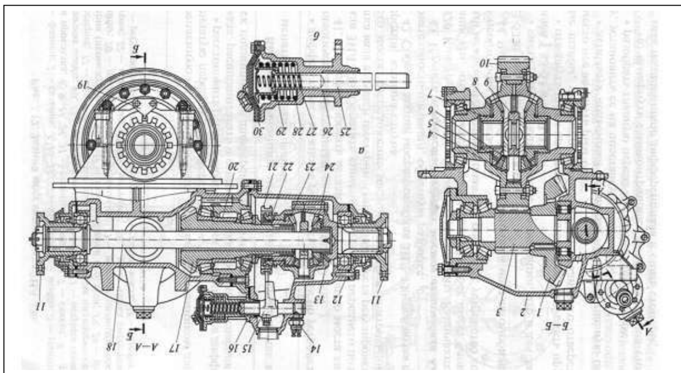
Рис. 3 Промежуточный мост автомобиля КамАЗ- 5320
