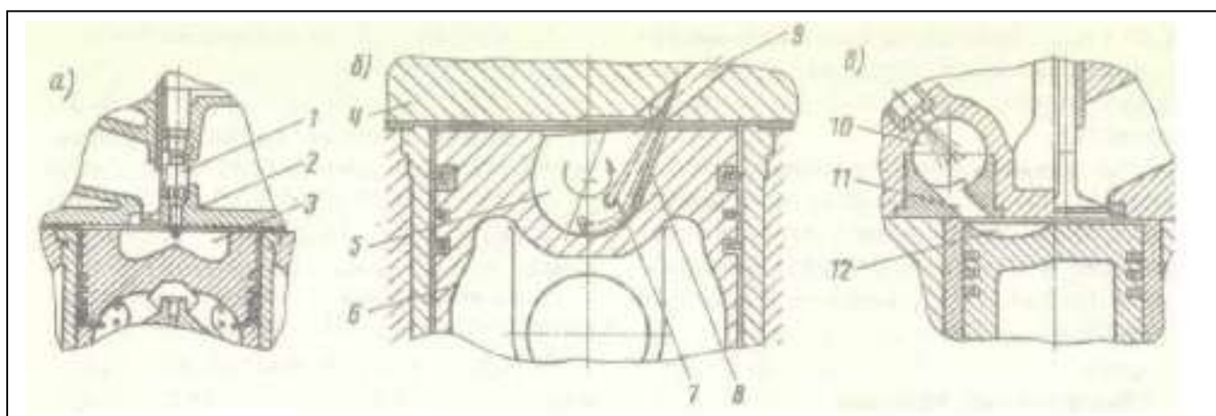
6 – поршень; 7 и 8 – объемная и пристеночная струя; 10 – дополнительная вихревая камера; 11 – канал.
