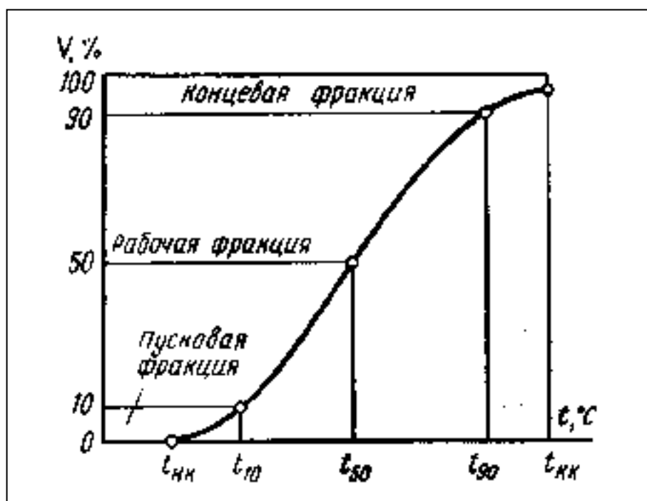
Рис. 5. Характерная кривая разгонки бензина.
