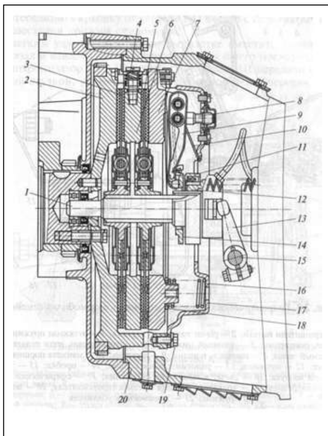
Рис..3. Сцепление в автомобилях семейства КамАЗ:
