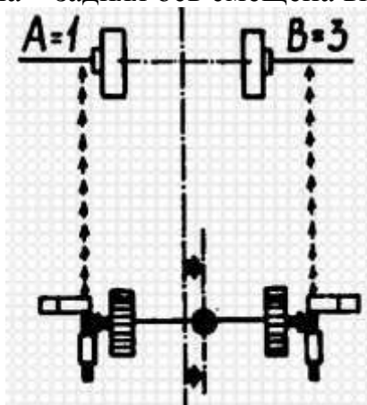
Рисунок 22 – Схема смещения задней оси вправо
