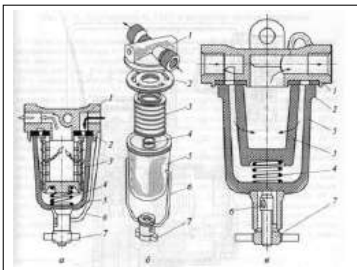
Рис. 7.3. Фильтры тонкой очистки топлива двигателей ЗМЗ-53 и ЗИЛ-130:
