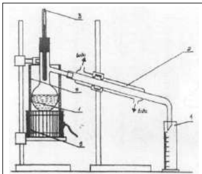
Рис. 3. Прибор для определения фракционного состава топлива:
