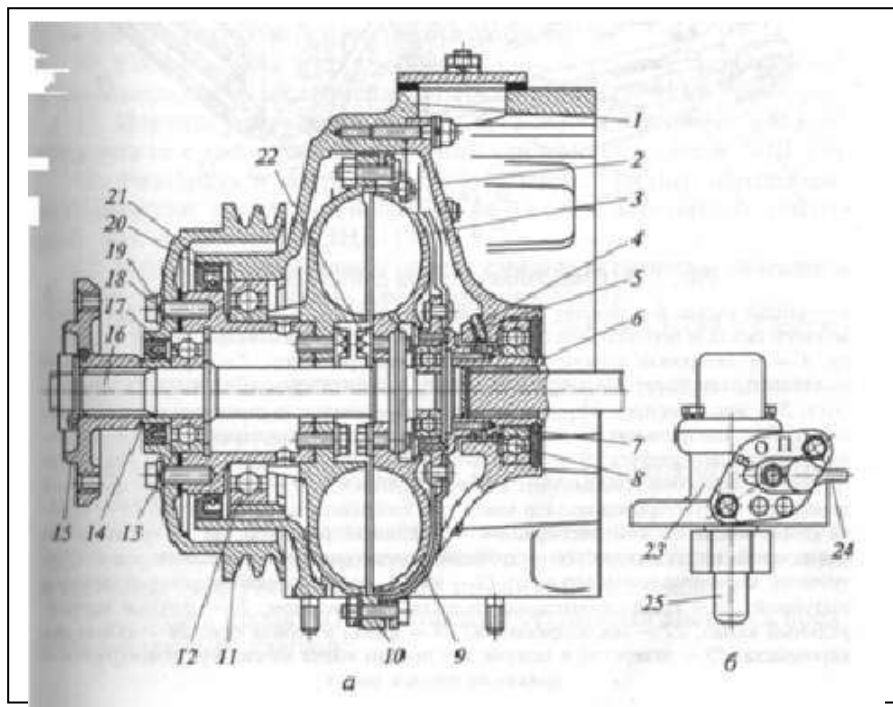
Рис. 5.5. Гидромукфа привода вентилятора двигателя КамАЗ-740:
