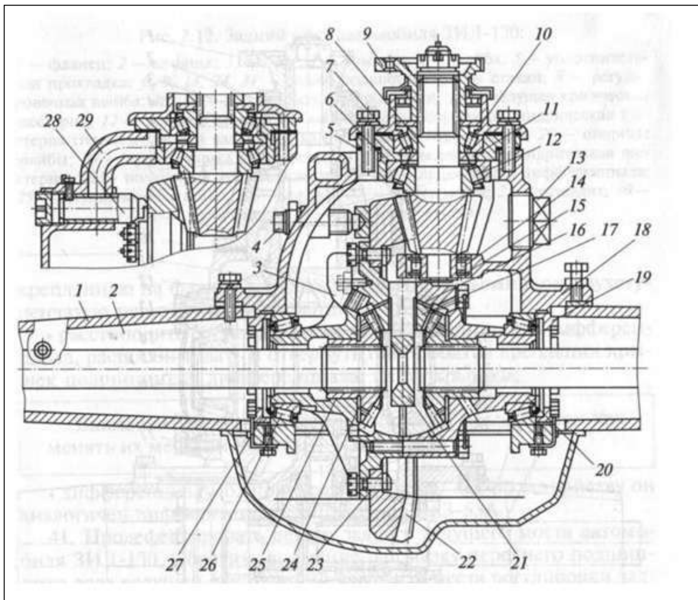
Рис. 1. Задний мост автомобиля ГАЗ-53А (ГАЗ-53-12):
