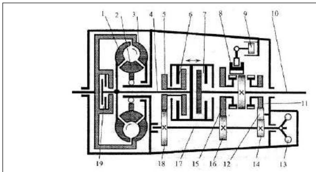
Рис. 2. Схема гидромеханической коробки передач:
