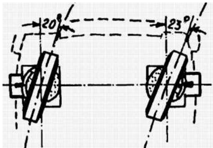
Рисунок 20 – Схема проверки рассогласования поворота колес
