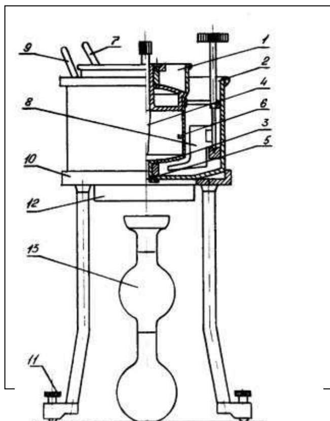
Рис. 15. Вискозиметр ВУ для определения условной вязкости масел:
