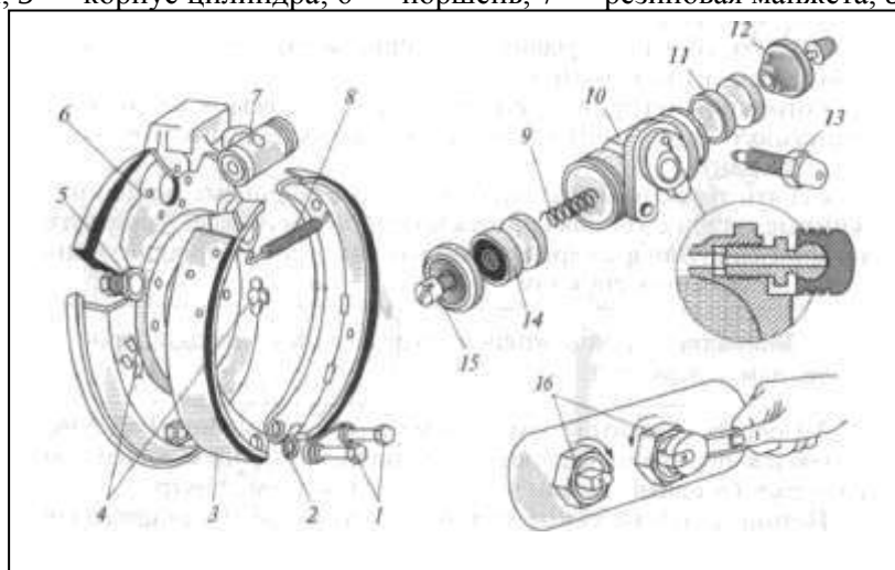
Рис. 3. Колесный тормозной механизм автомобиля ГАЗ-53А:
