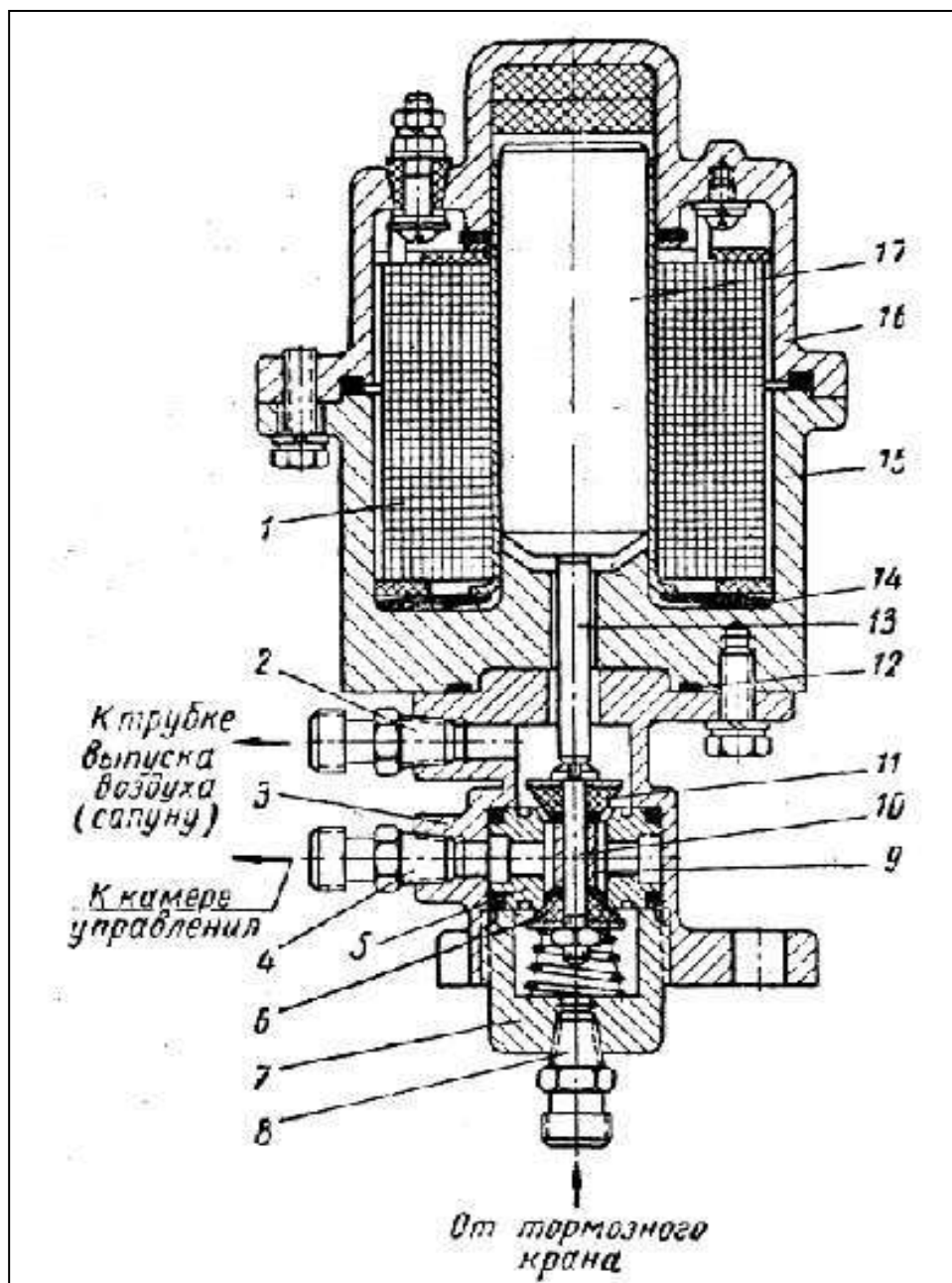
Рисунок 2 □ Электромагнитный клапан управления: 1– электромагнит; 2– штуцер выпуска воздуха; 3 – корпус клапана управления раздаточной коробкой; 4 – штуцер; 5 – седло клапана; 6 – впускной клапан; 7 – пробка клапана; 8 – штуцер; 9 – распорная втулка; 10 – стержень клапана; 11 – выпускной клапан; 12–уплотнительное кольцо; 13 – шток; 14 – дисковая пружина; 15 – корпус; 16 – крышка; 17 – сердечник.
