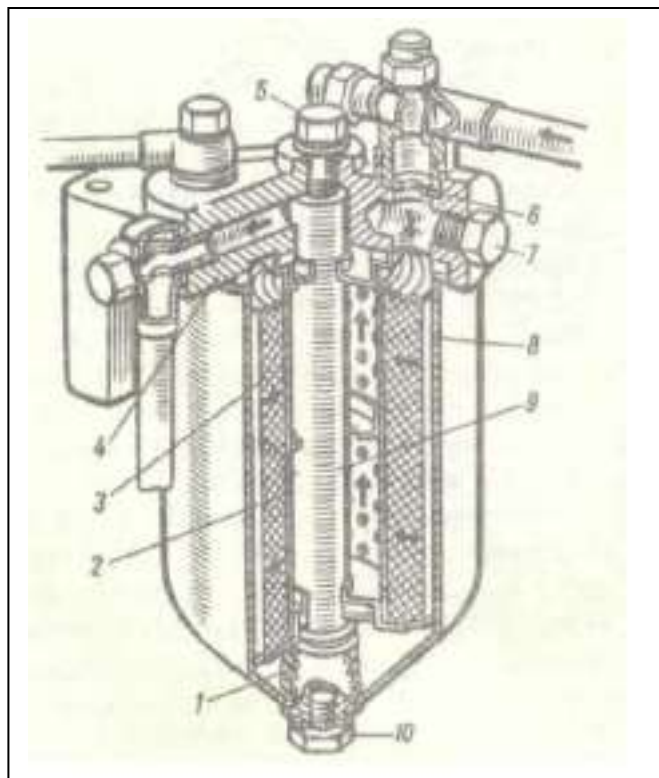
Рисунок 3 - Фильтр тонкой очистки топлива
