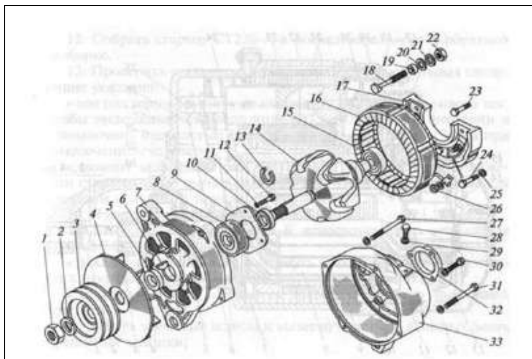
Рис. 12.3. Схема разборки генераторной установки Г237-В:
