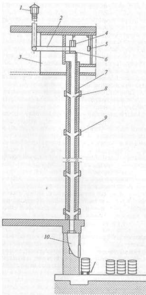
Рис. 1. Схема мусоропровода:
