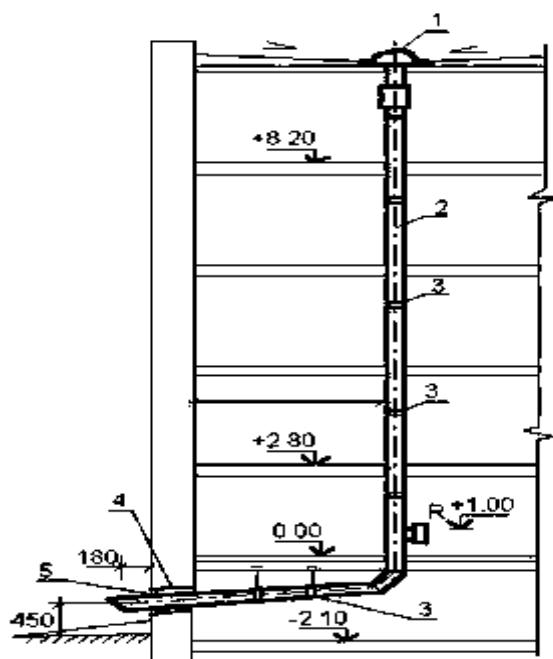
Рис. 7.1. Схема внутреннего водостока: 1 – воронка; 2 – водосточный стояк; 3 – крепления стояка и выпуска; 4 – гильза, зачеканенная смоляной прядью; 5 – цементная штукатурка.
