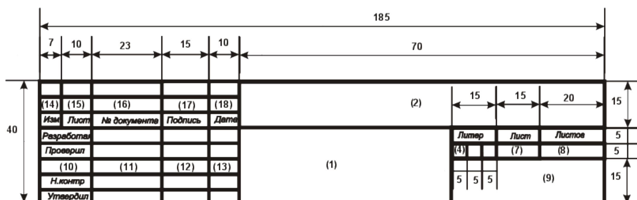
Рисунок 3 – Основная надпись на первом листе спецификации
