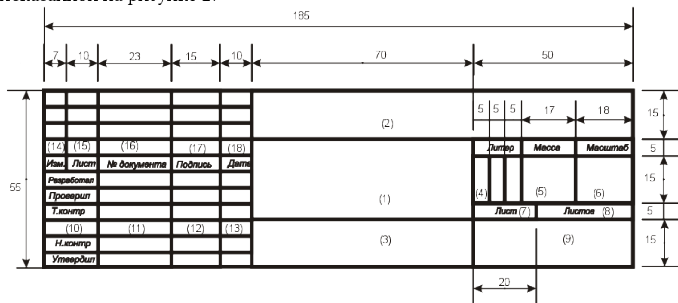
Рисунок 2 - Основная надпись на чертежах
