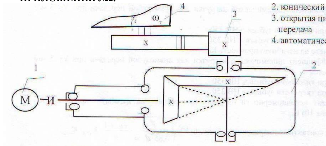
Схема привода
