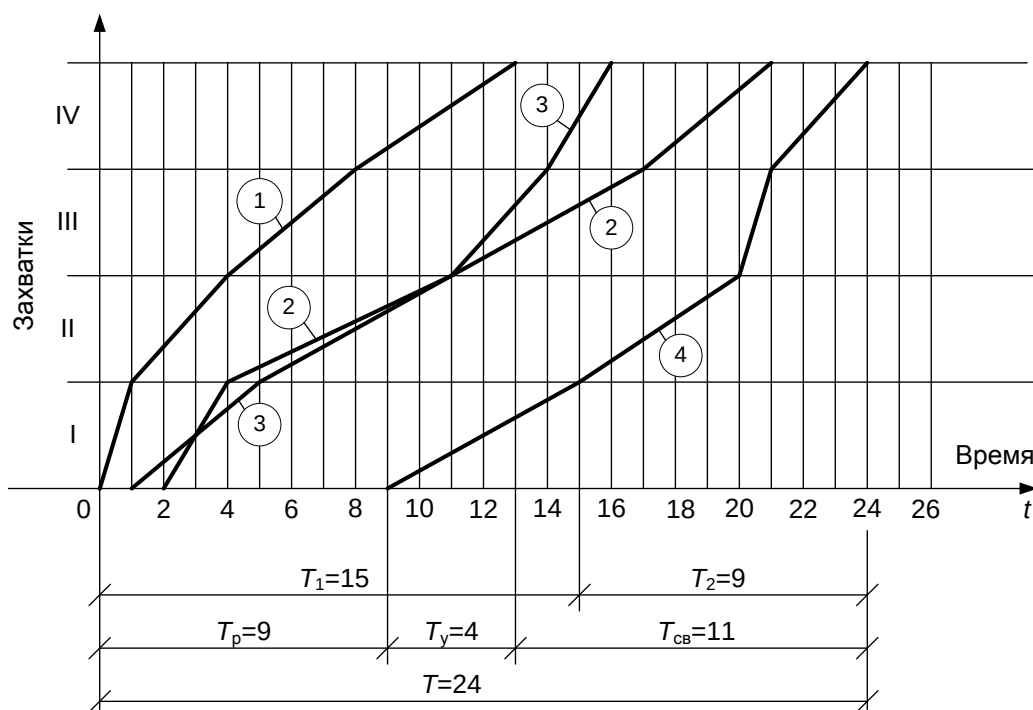
Рисунок 3.7 Модель неритмичного потока в виде циклограммы с совмещением процессов
