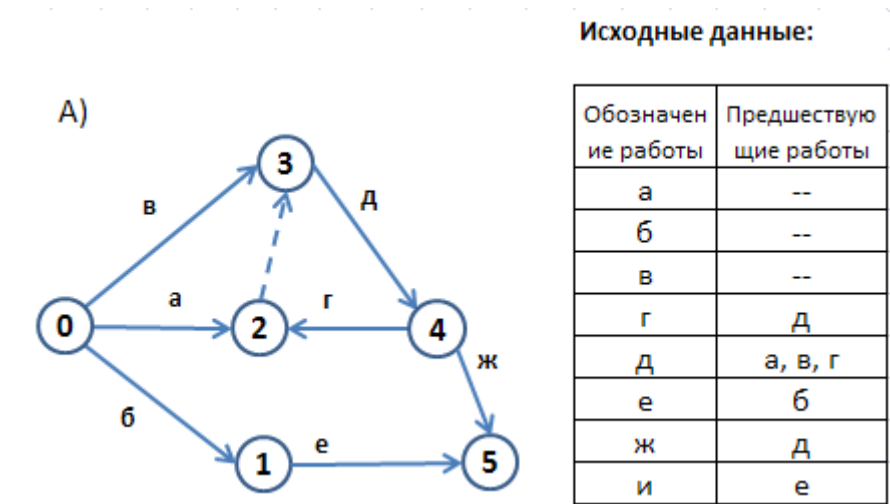
Рис. 10 (А). Пример цикла на сетевом графике
