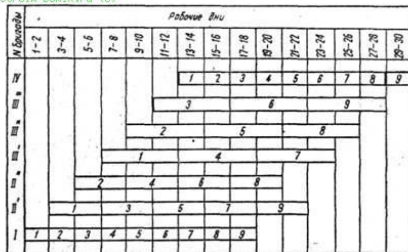
Рис. 4. График производства работ поточным методом с кратным ритмом два, четыре и шесть дней
