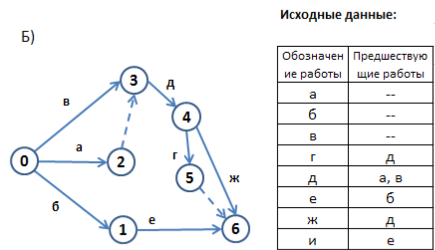
Рис. 10 (Б). Устранение цикла на сетевом графике
