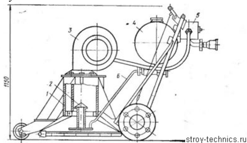
Рис. 174. Машина СО-107 для сушки оснований кровли 1 — камера сгорания; 2 — горелка; 3 — вентилятор; 4 — топливная система; 5 — электрооборудование; 6 — топливопровод
