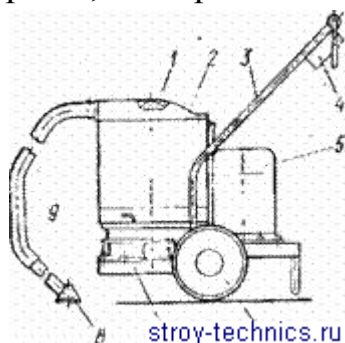
Рис. 173. Машина СО-106 для удаления воды с основания кровли 1 — крышка; 2 — водосборный бак; 3 — ручка; 4 — электрооборудование; 5 — г-электродвигатель; 6 — колесо; 7 — рама; 8 — насадка; 9 — воздуходувка Машина проста в обслуживании, маневренна. Наледь удаляется открытым пламенем, а сушка основания кровли осуществляется инфракрасным излучением.
