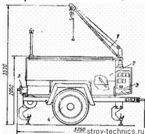
Рис. 183. Установка для варки битума передвижная УБВ-3 1 — кран-укосина; 2 — емкость; 3 — пульт управления; 4 — шасси; 5 — слив
