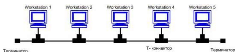
Рисунок 1 – Шинная топология
