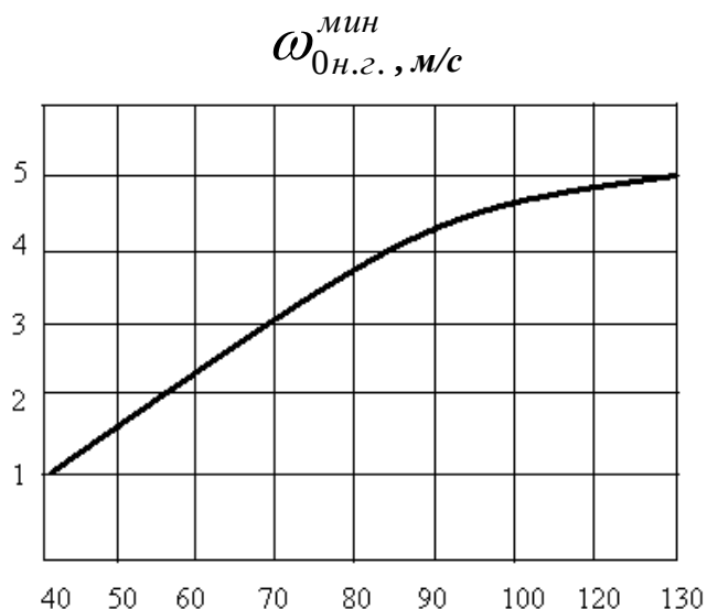
Рисунок 6.8 - Зависимость скорости проскока от диаметра носика горелки
