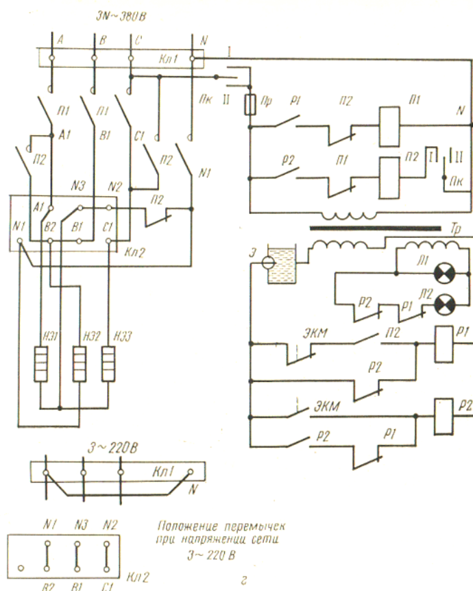
Рисунок 8.1 – Принципиальная электрическая схемы пищеварочного котла.
