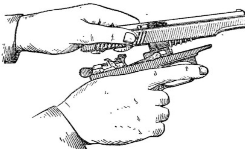
Рис. 6. Введение свободного конца возвратной пружины в канал затвора чтобы дульная часть ствола прошла через канал затвора и выступила наружу (рис. 7). Опустить задний конец затвора на рамку так, чтобы продольные выступы затвора поместились в пазах рамки, и, прижимая затвор к рамке, отпустить его. Затвор под действием возвратной пружины энергично возвращается в переднее положение. Включить предохранитель (поднять флажок вверх).
