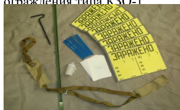
Комплект носимых знаков ограждения типа КЗО-1
