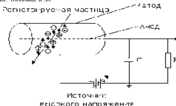
Рисунок 2. 4 – Принципиальная схема конструкции ГС
