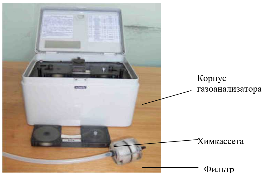
Рисунок 3.2 – Общий вид газоанализатора ГАНК-4
