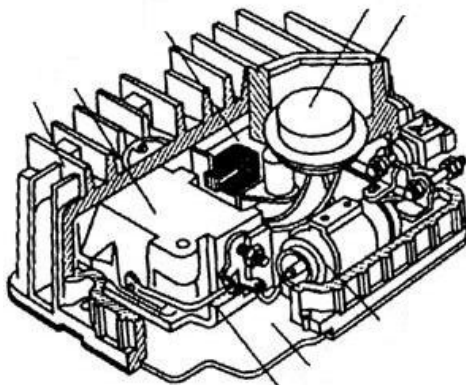
Рис. 2. Электронный коммутатор:
