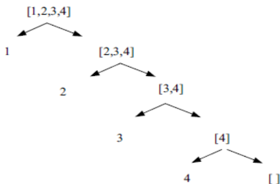
Рисунок 4.1 - Бинарное дерево списка.
