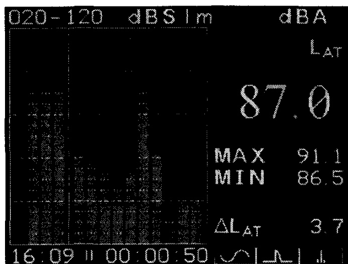
Рисунок 7 - Индикация в режиме dBSlm
