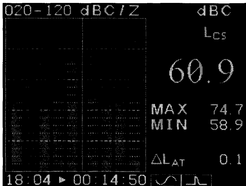
Рисунок 14 - Индикация в режиме dBc/Z.
