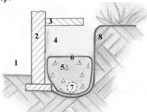
Рис. 1. Схема устройства пристенного дренажа
