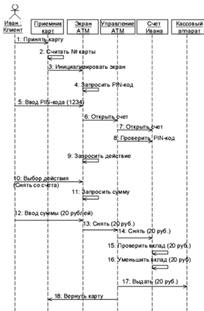
Рисунок 2.7 - Пример диаграммы последовательности
