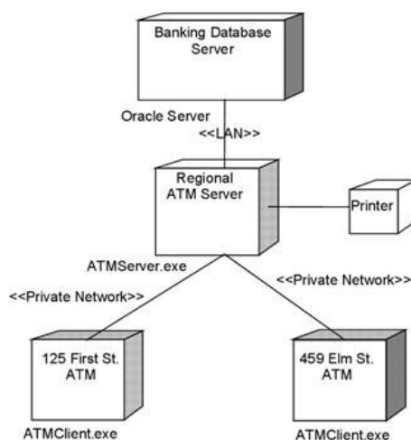
Рисунок 2.19 - Пример диаграммы размещения
