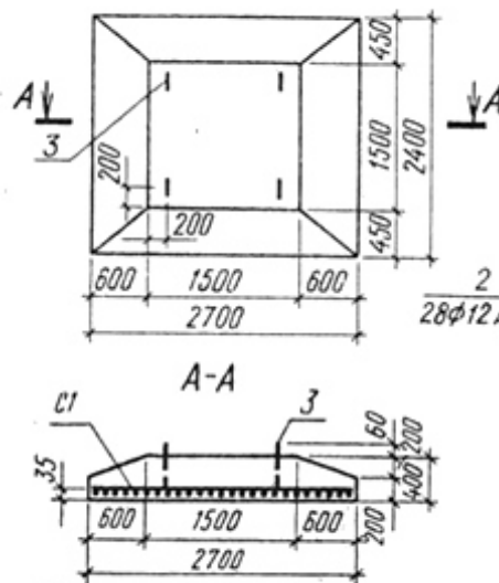
Фундаментная подушка
