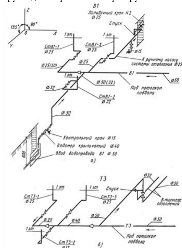
Рис. 18.3 Аксонометрическая схема
