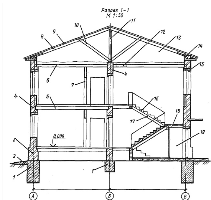
Рис. 4.1. Конструктивные элементы здания с несущими стенами:
