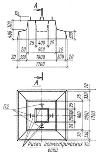
Фундамент
