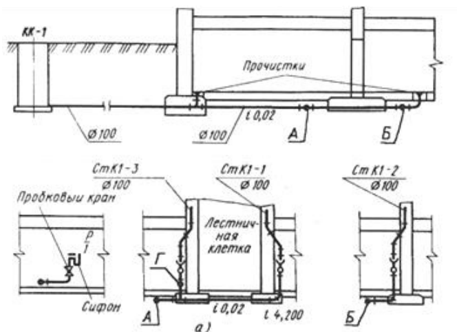
Рис 18.5 Фрагмент монтажного плана санитарного узла.
