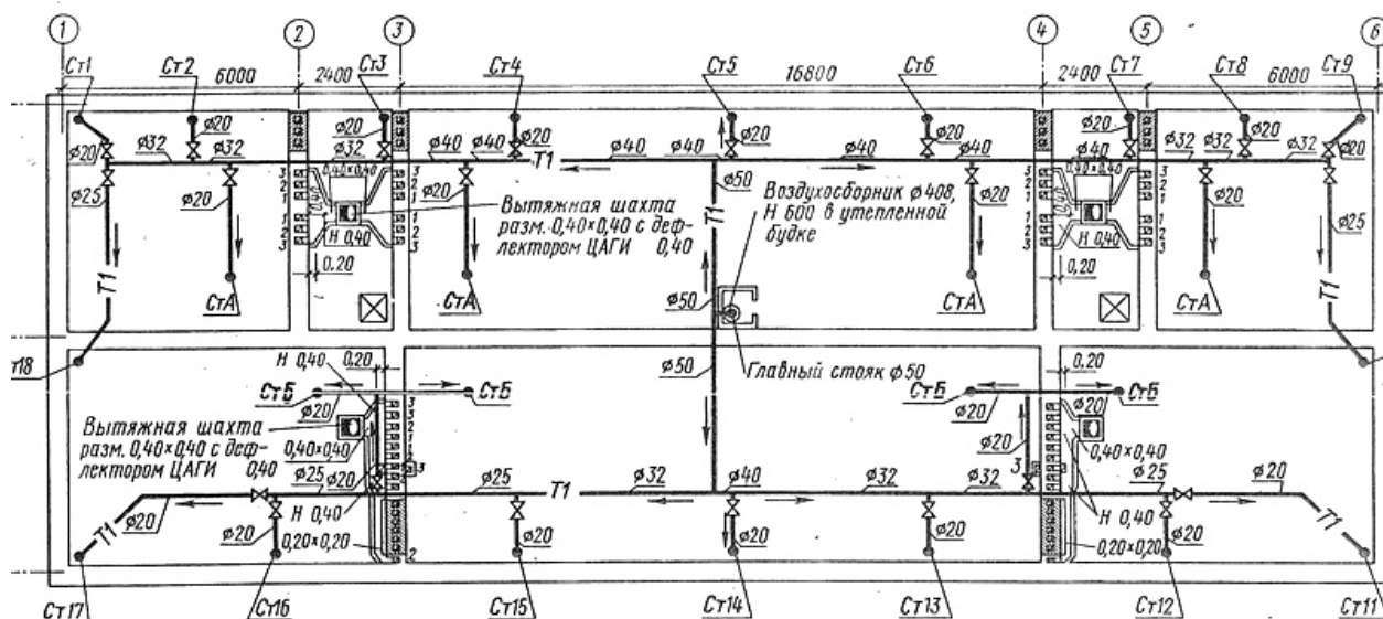
План чердака
