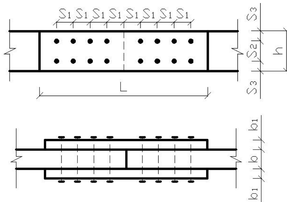
Рис.11. Нагельное соединение двух брусев накладками
