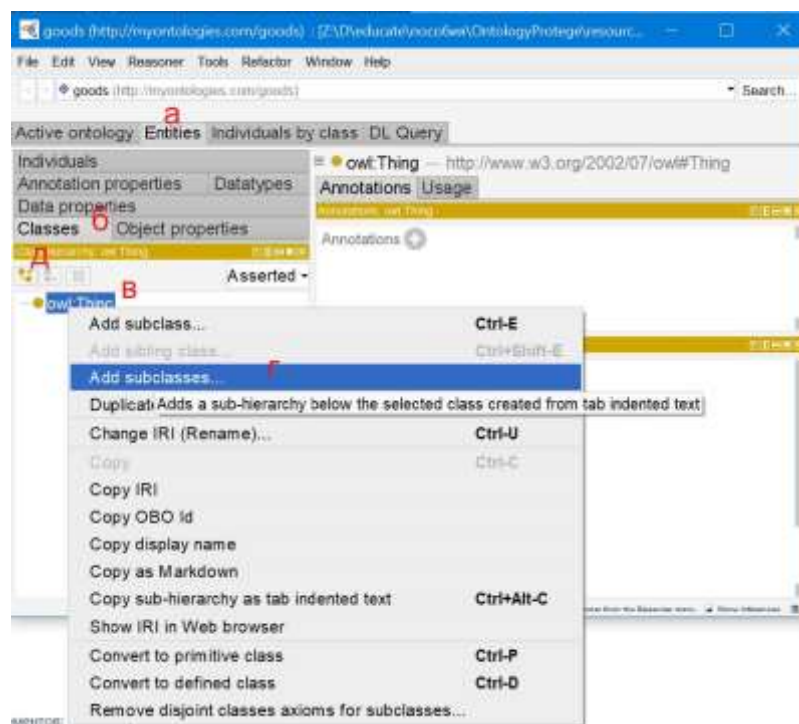
Рис. 5 Вкладка «Entities» в системе Protégé (а – панель в вкладку с активной вкладкой «Entities»; б – панель вложенных вкладок вкладки «Entities» с активной вкладкой «Classes»; в – суперкласс owl:Thing; г, д – кнопки добавления иерархии подклассов/подкласса для выделенного класса)
