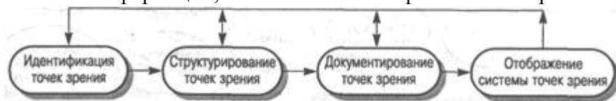
Рисунок 1.3 - Метод VORD
