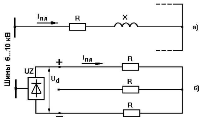
Рисунок 1.1 - Принципиальные схемы плавки гололеда переменным (а) и постоянным (б) током
