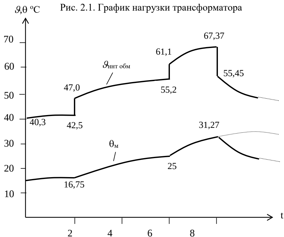
Рис. 2.2. Изменение температуры наиболее нагретой точки обмотки трансформатора Максимальная температура наиболее нагретой точки в конце третьей ступени нагрузки \theta_{ннт\ max} = 20+31,27+16,1 = 67,37^{\circ}C .
