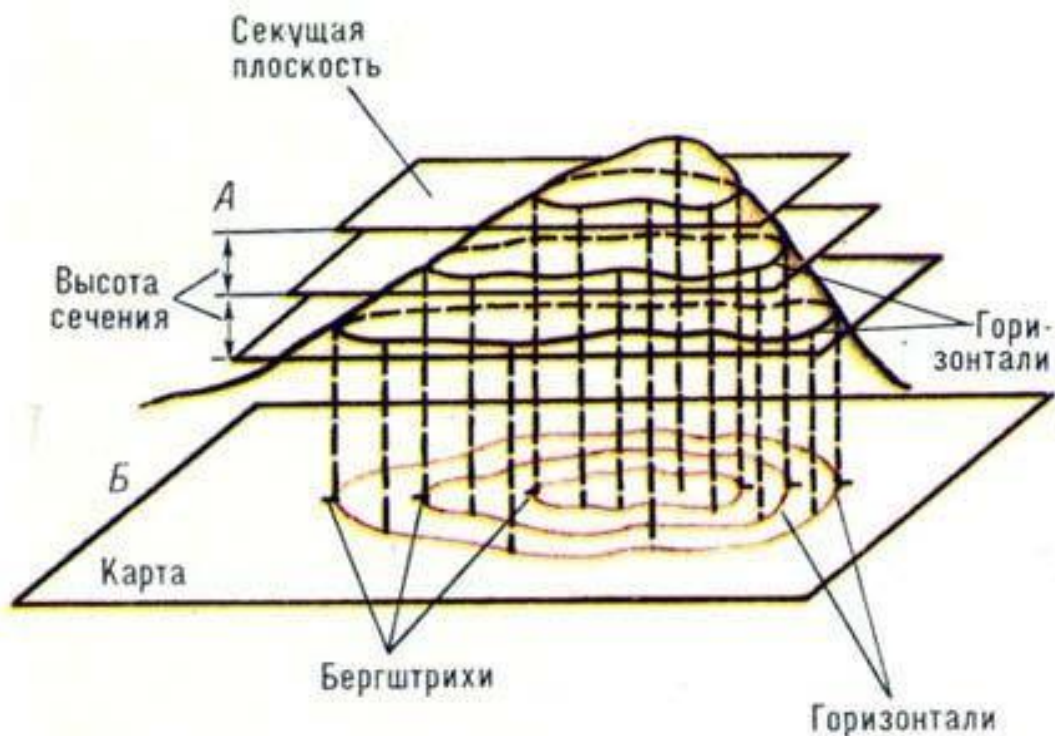
Рисунок 1 - Принцип получения горизонталей и проектирование их на
