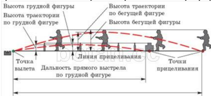
Рис. 51. Прямой выстрел
