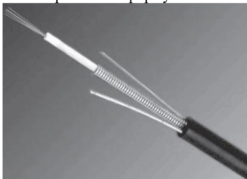
Рис. 5. Оптоволоконный кабель
