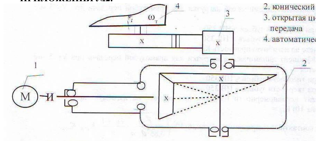
Схема привода
