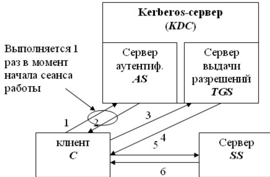
Рис. 4.1. Протокол Kerberos
