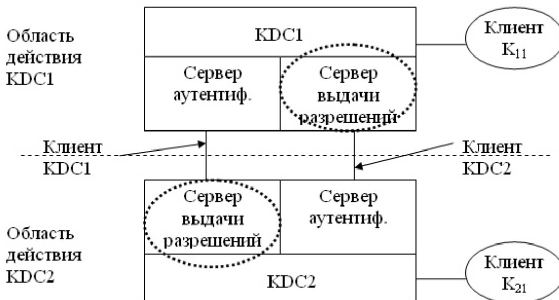
Рис. 4.2. Взаимодействие между Kerberos-областями
