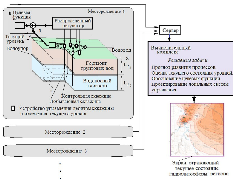
Рис.1.1. Сеть мониторинга и управления гидролитосферными процессами региона .
