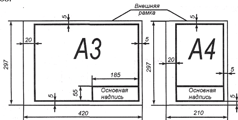
Рисунок 1. Примеры размеров сторон форматов A4 и A3
