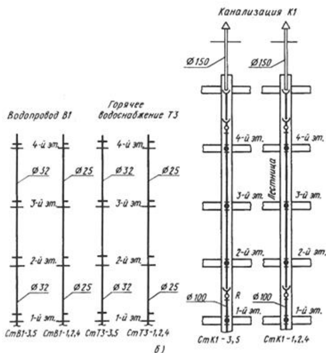
Рис. 18.5 Фрагмент монтажного плана санитарного узла.
