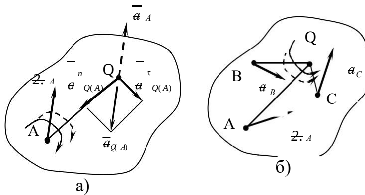
Рисунок 11. Определение мгновенного центра ускорений.
