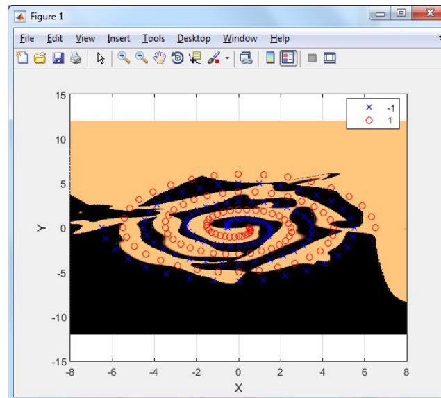
Рисунок 5.23 – Полученная поверхность отклика для пользовательской сети
