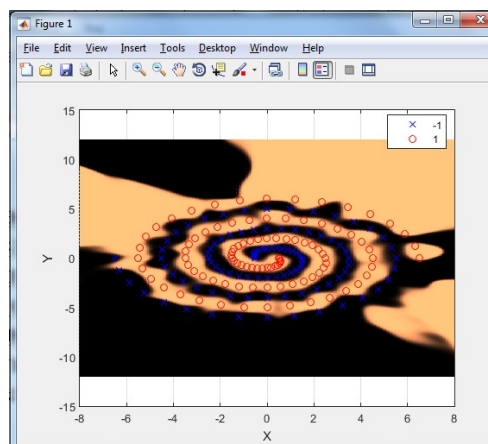
Рисунок 5.17– Поверхность отклика после применения алгоритма trainlm
