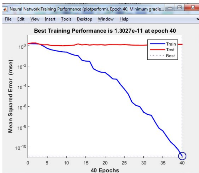
Рисунок 5.16 – Ошибка обучения и обобщения для 40 эпох
