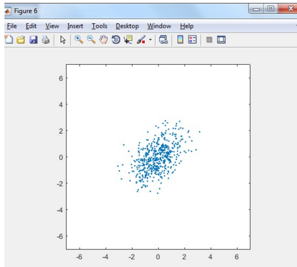
Рисунок 1.7 – Сгенерированное множество точек для случая \mu_1^2 = 0.2, \mu_2^2 = 1, \mu_{12} = 0.5
