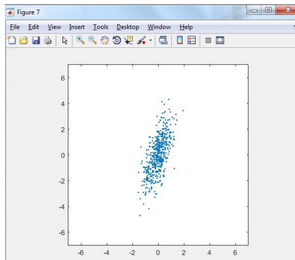
Рисунок 1.8 – Сгенерированное множество точек для случая \mu_1^2 = 0.3, \mu_2^2 = 0.5, \mu_{12} = 0.2
