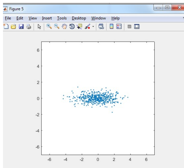
Рисунок 1.6 – Сгенерированное множество точек для случая \begin{matrix} ? \\ 1 \end{matrix}^2 \bullet 2, \begin{matrix} ? \\ 2 \end{matrix}^2 \bullet 0.2, ? \bullet 0
