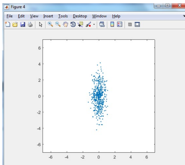
Рисунок 1.5 – Сгенерированное множество точек для случая \begin{matrix} ? \\ 1 \end{matrix}^2 \bullet 0.2, \begin{matrix} ? \\ 2 \end{matrix}^2 \bullet 2, ? \bullet 0
