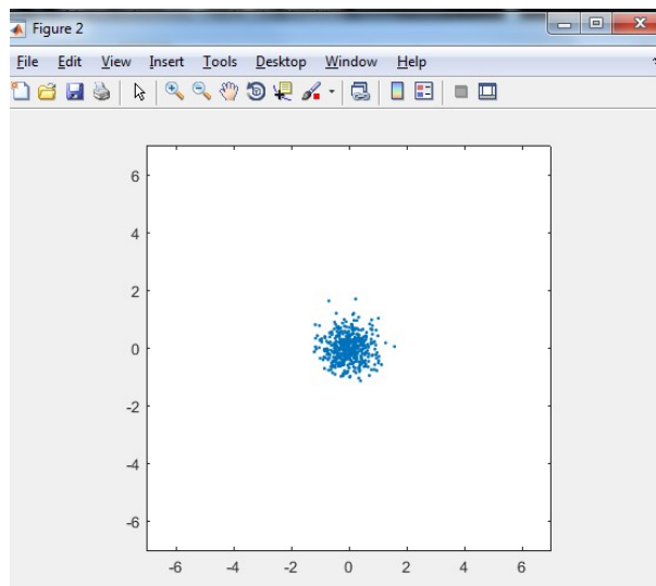
Рисунок 1.3 – Сгенерированное множество точек для случая \begin{matrix} ? & \bullet & ? \\ 1 & 2 & 12 \end{matrix}^2 \bullet 0.2, \quad ? \bullet 0
