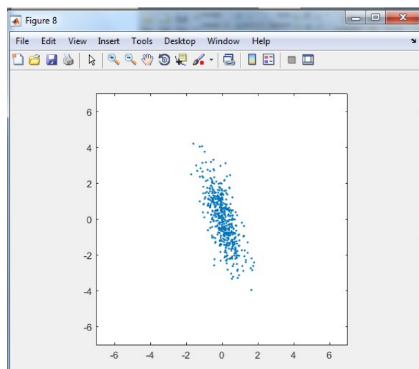
Рисунок 1.9 – Сгенерированное множество точек для случая \mu_1^2 = 0.3, \mu_2^2 = 0.5, \mu_{12} = 0.2
