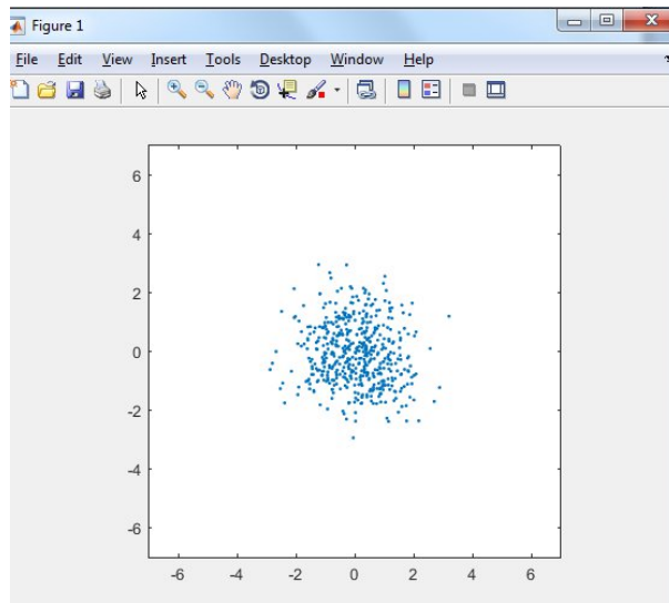
Рисунок 1.2 – Сгенерированное множество точек для случая \begin{matrix} ? & \bullet & ? \\ 1 & 2 & 12 \end{matrix}^2 \bullet 1, \quad ? \bullet 0
