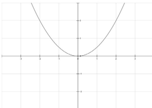
Рисунок 1. Функция y=x^2
