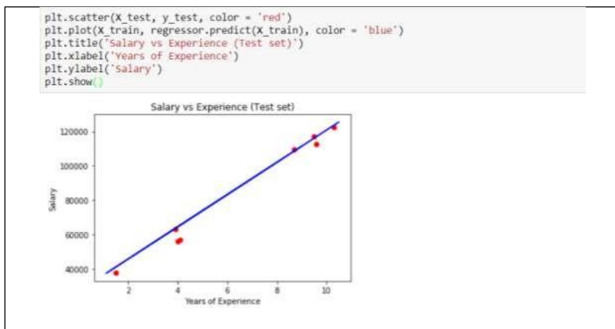
Рисунок 8.1 – Код Python, отражающий общий пайплайн для задачи одномерной регрессии
