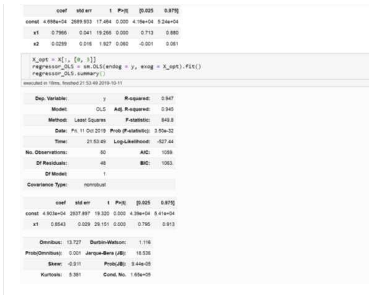
Рисунок 9.2 – Оптимизация модели многомерной регрессии
