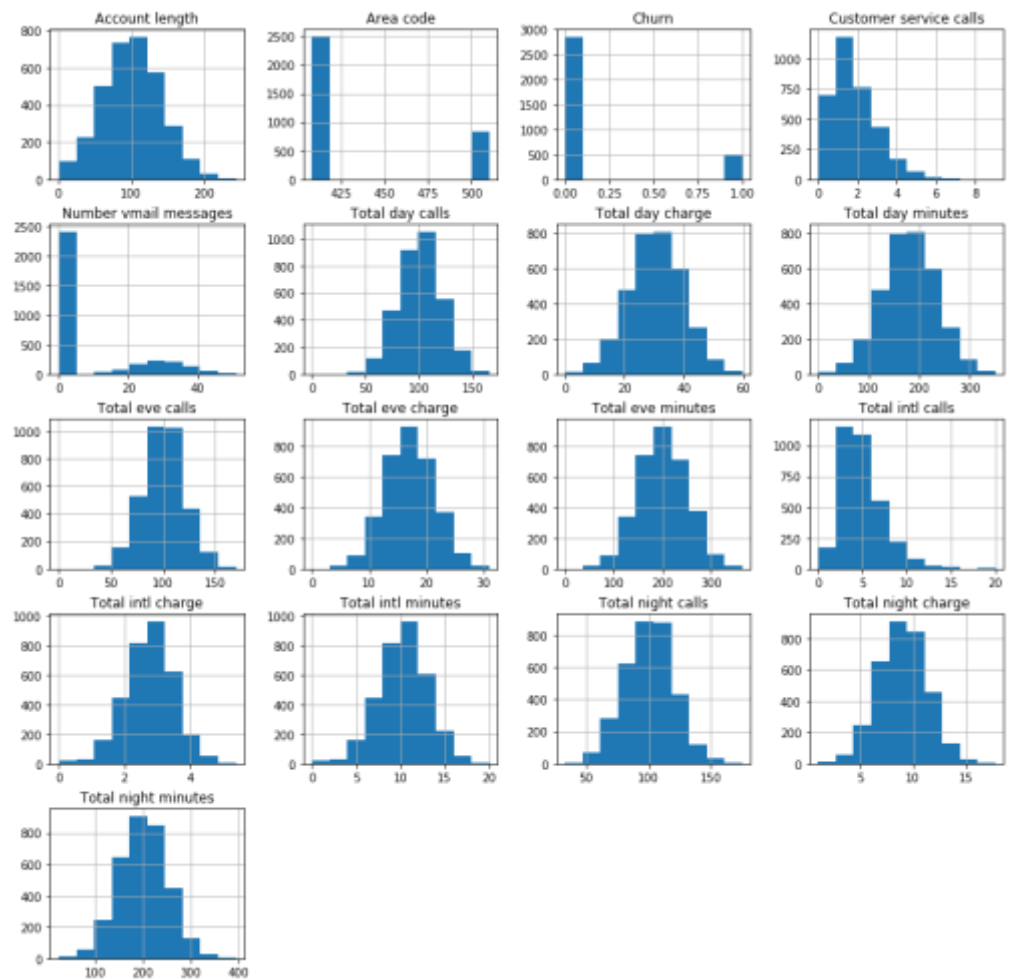
Рисунок 2.4 – Применение метода hist() для визуализации распределения нескольких признаков
