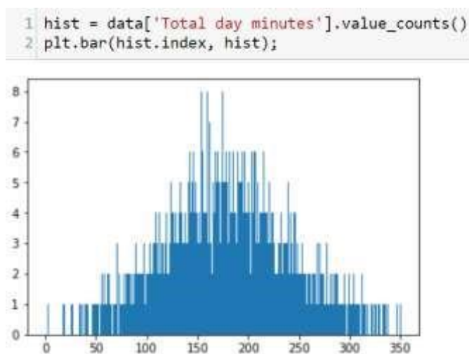
Рисунок 2.6 – Использование matplotlib для представления распределения значений признака
