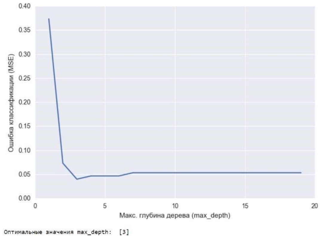
Рисунок 4.4 – Вывод зависимости значения MSE от параметра max_depth
