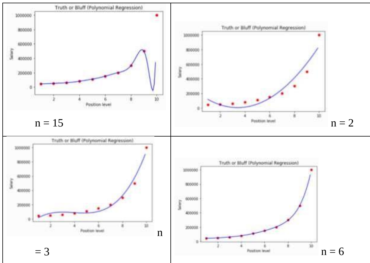
Рисунок 10.2 – Анализ модели полиномиальной регрессии
