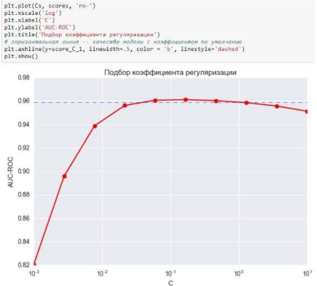
Рисунок 5.18 – График зависимости AUC-ROC от гиперпараметра
