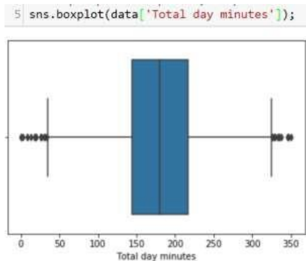
Рисунок 2.7 – График «ящик с усами» для отдельного признака
