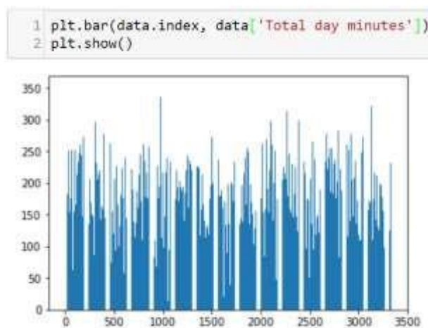
Рисунок 2.5 – Построение гистограммы с использованием matplotlib
