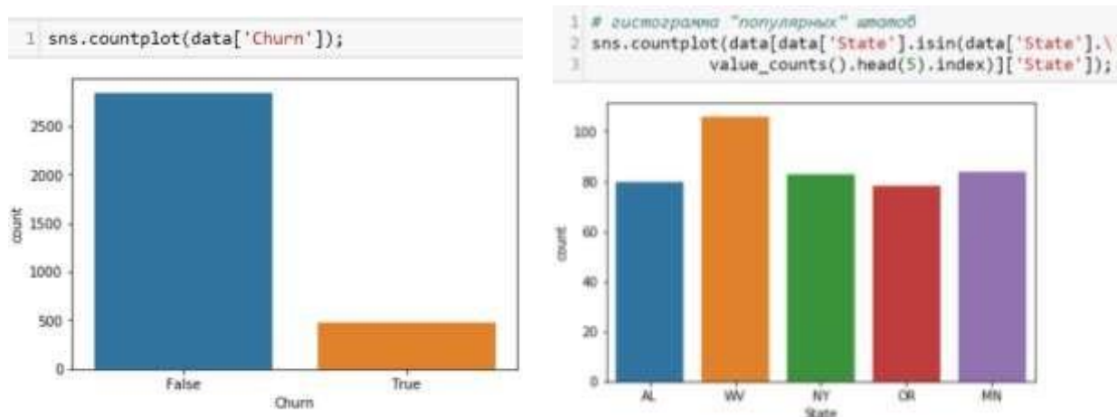
Рисунок 2.10 – График countplot: а) визуализация распределения признака Churn; б) визуализация пяти популярных штатов
