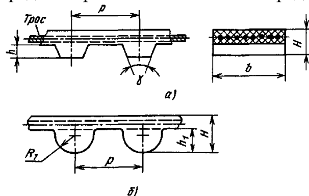
Рисунок 5.5 – Зубчатые ремни
