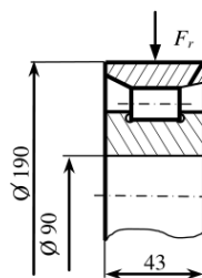
Рисунок 8.1 – Эскиз подшипника
