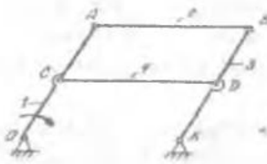
Рисунок 1.12 – Схема механизма с пассивной связью
