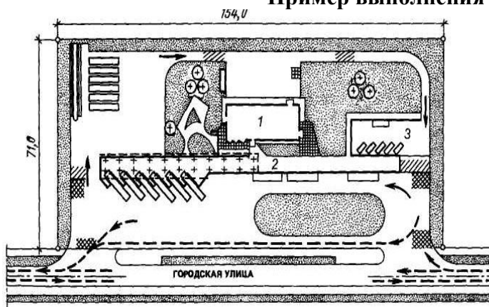
Рис. 12. Пример графического оформления чертежа плана благоустройства территории: 1 — промышленное здание, 2 — проходная, 3 — автостоянка
