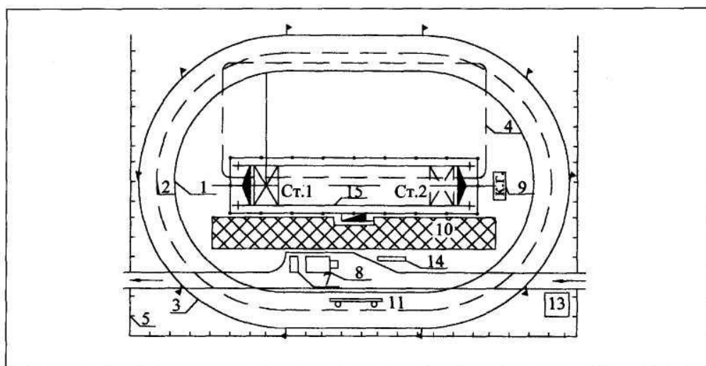
Рис. 14. Пример выполнения чертежа стройгенплана
