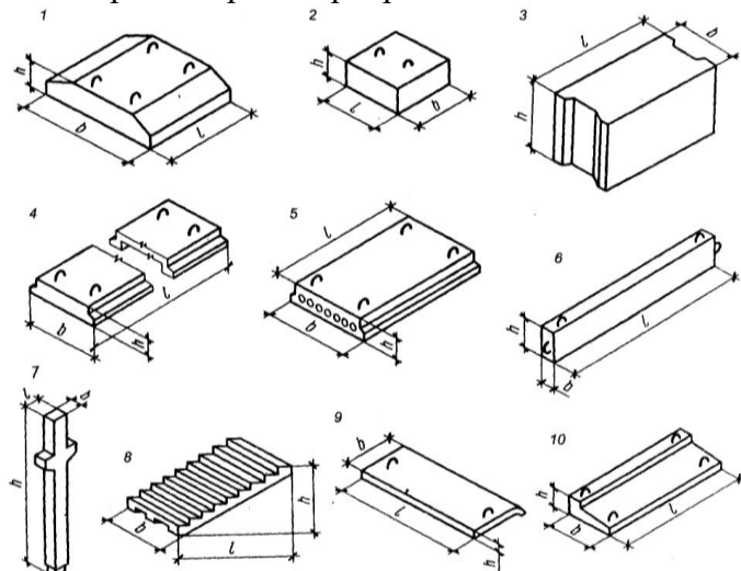
Рис. 10. Эскизы бетонных конструкций
