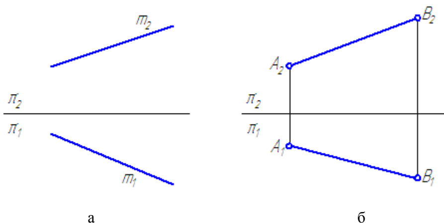
Рисунок 4 – Проекции прямой
