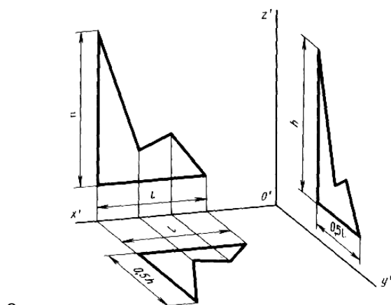
Рисунок 9 диметрии диметрии
