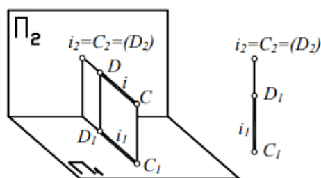
Рис. 12. Фронтально-проецирующая прямая
