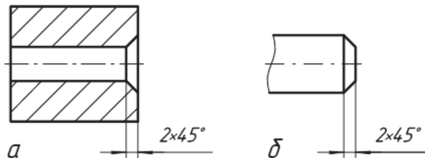
Рис. 31. Обозначение фаски
