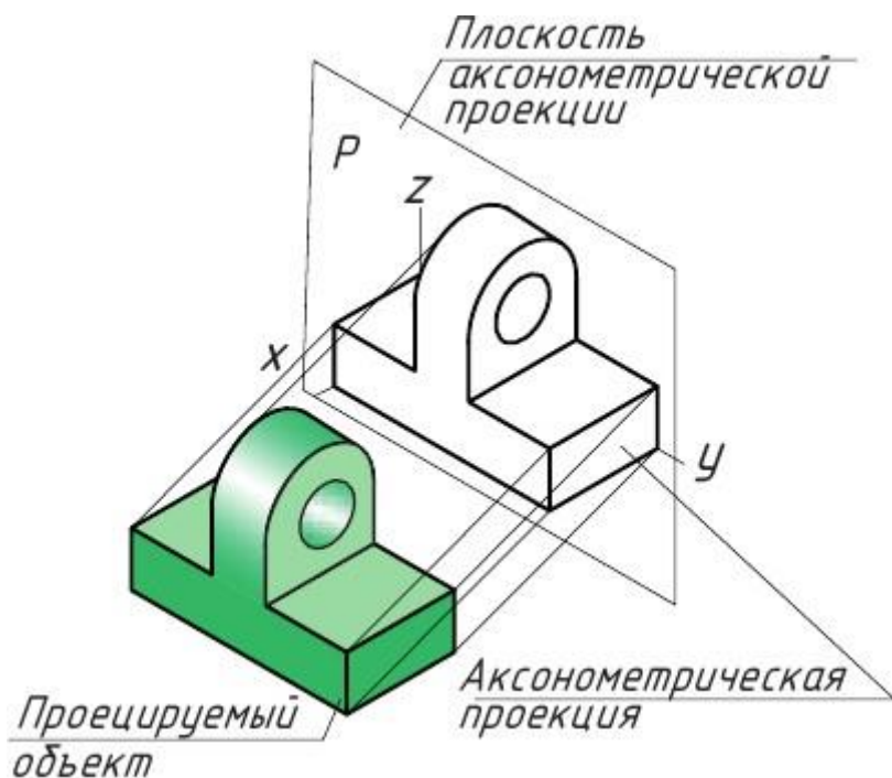
Рис. 54. Аксонометрическая проекция
