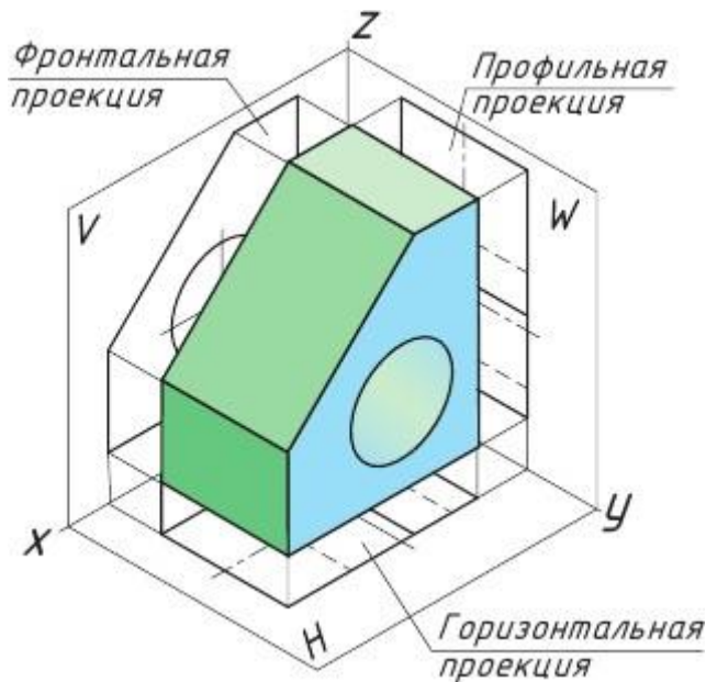
Рис. 49. Комплексный чертеж
