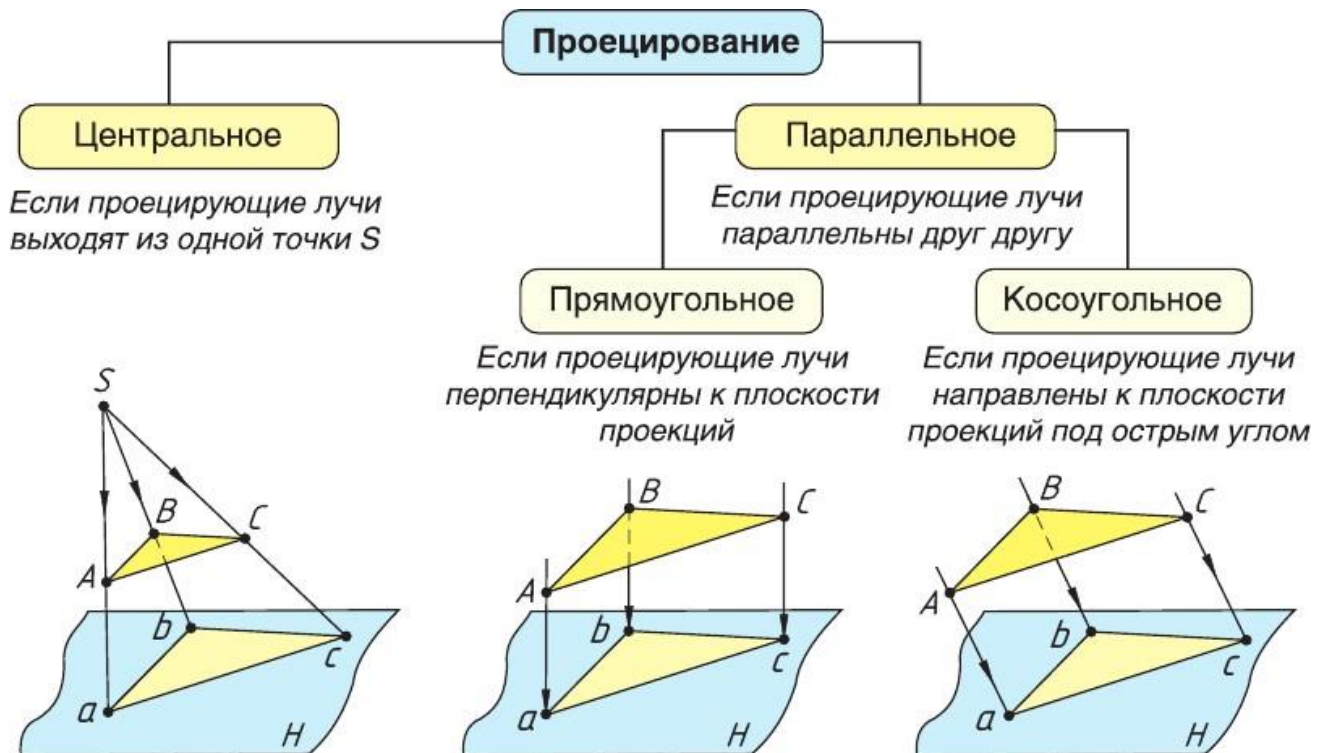
Рис. 40. Виды проецирования
